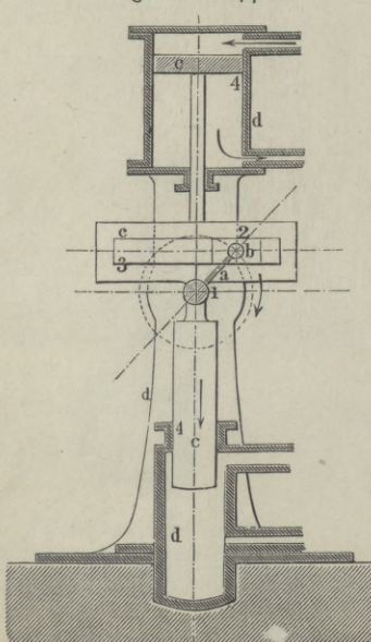
Fig. 2. Dampfsm.
