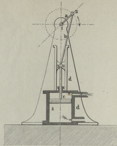
Fig. 1. Dpfm. Pumpe.
