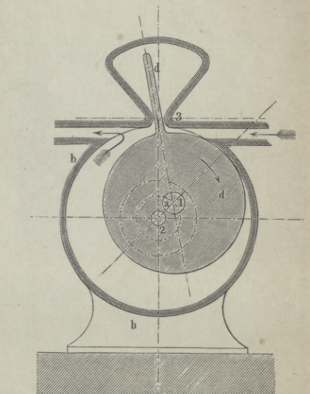
Fig. 14. Wedding, Gebläse.
