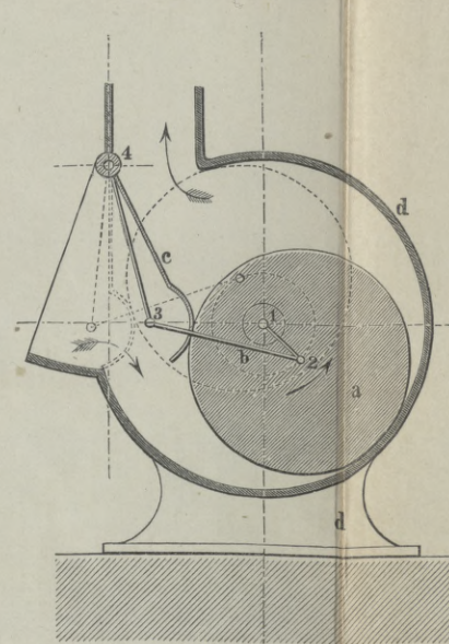
Fig. 12. Cooke. Gebläse.
