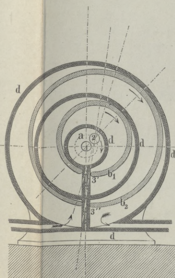
Fig. 6. Lamb, Dpfm.
