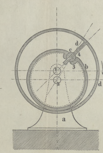
Fig. 17. Cochrane. Dpfm.
