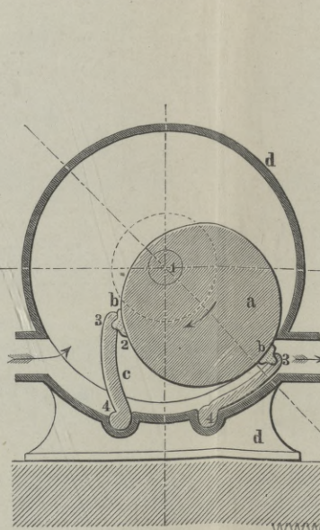
Fig. 10. Dundonald. Dpfm.
