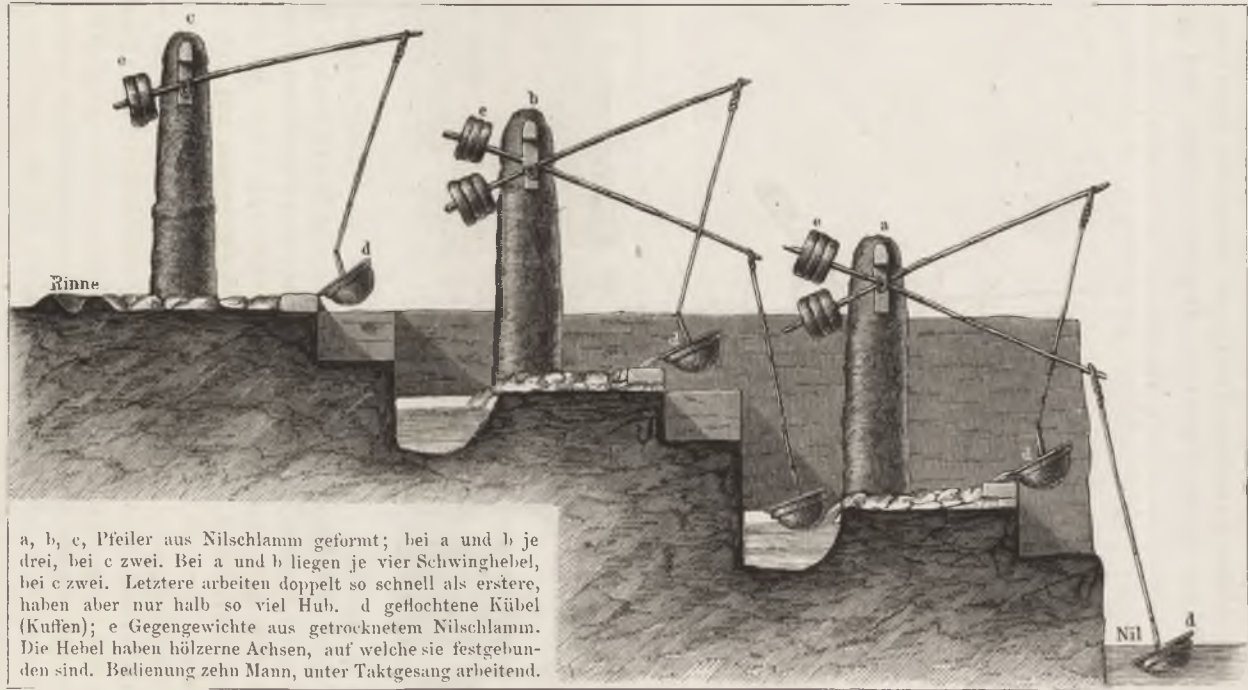
Fig. 171. Aegyptische Schaduff-Anlage.
