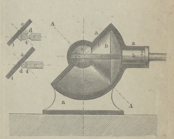
Fig. 12. Geiss. Dpfm.
