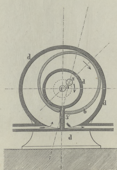
Fig. 5. Lamb, Dpfm.
