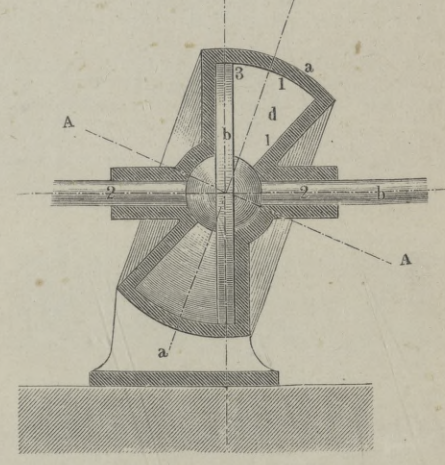
Fig. 9. Duclos. Dpfm.
