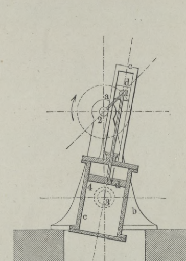
Fig. 9. Murdock, Dpfm.
