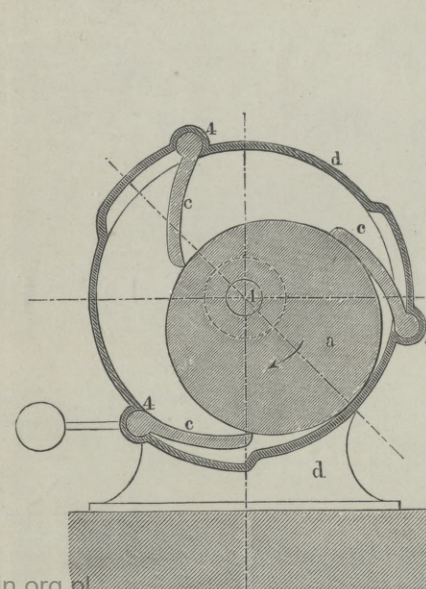
Fig. 11. Cochrane. Dpfm.
