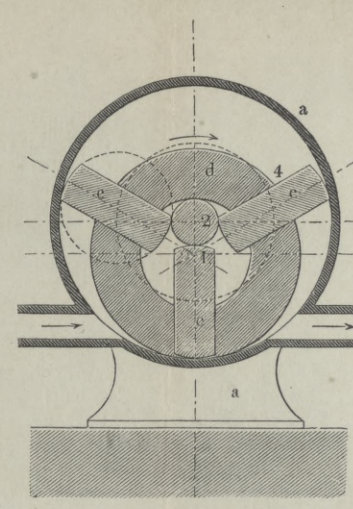
Fig. 8. Jones. Ortlieb. Dpfm. Pumpe.
