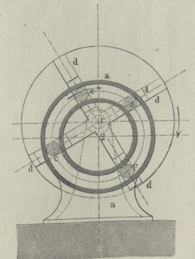
Fig. 10. Smyth. Dpfm.
