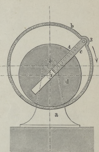
Fig. 4. Cochrane. Dpfm.
