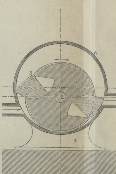
Fig. 16. Cochrane. Dpfm.
