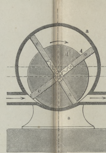
Fig. 7. Ramelli. Pumpe.
