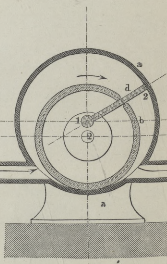
Fig. 13. Cochrane. Dpfm.
