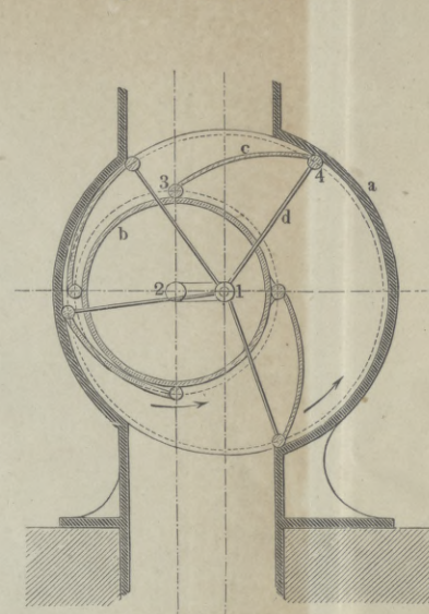
Fig. 14. Lemielle. Gebläse.
