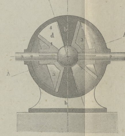
Fig. 5. Duncan. Dpfm.
