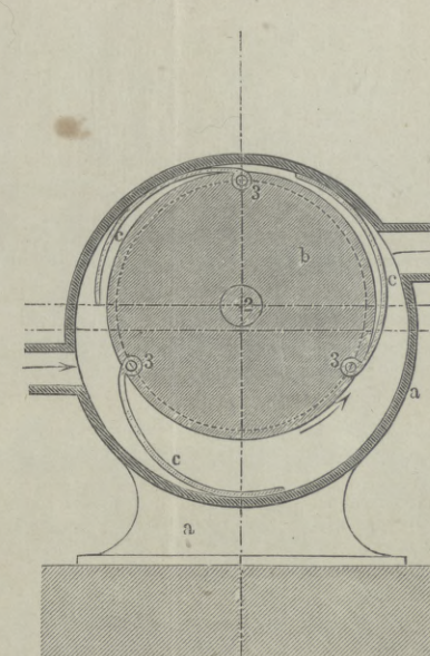
Fig. 15. Ramelli. Pumpe.
