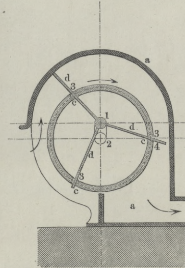
Fig. 12. Bellford. Gebläse.
