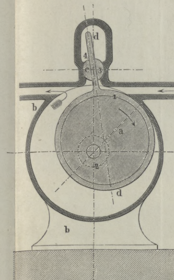
Fig. 13. Knott, Pumpe.
