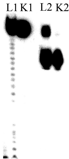
Rysunek 61. Ograniczona hydroliza jonami Mg^{2+} w formamidzie: substratu (L1) oraz zcyrkularyzowanego oligomeru (L2). Literą K zaznaczono odpowiednio linie kontrolne.
