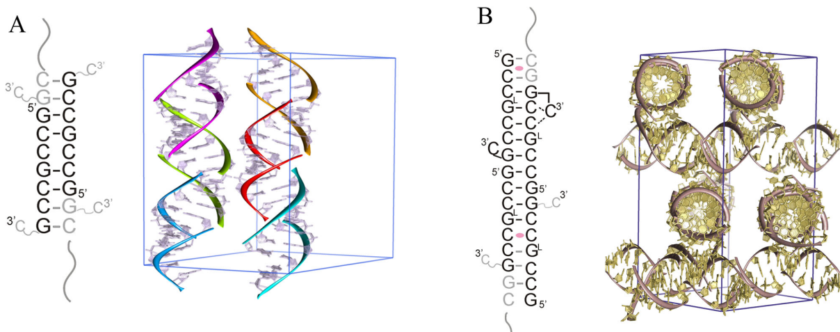
Rysunek 48. Struktura drugorzędowa oraz upakowanie cząsteczek w sieci krystalicznej struktury romboedrycznej (niemodyfikowanej) (A) oraz tetragonalnej (modyfikowanej) (B). Szarym zaznaczono nici symetryczne oraz nieuporządkowane reszty 8C. Krystalograficzna oś dwukrotna zaznaczona jest na różowo.
