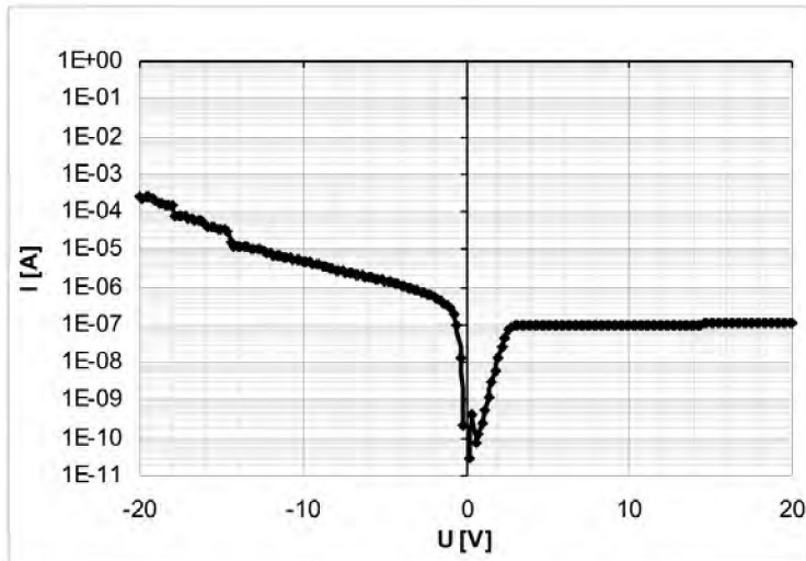
Fig. 3. Typical current voltage ( I - V ) characteristic of Al/BT/Si ( MIS ) structures. Fig. 3. Typowe charakterystyki prądowo-napięciowe ( I - V ) struktur Al/BT/Si.
