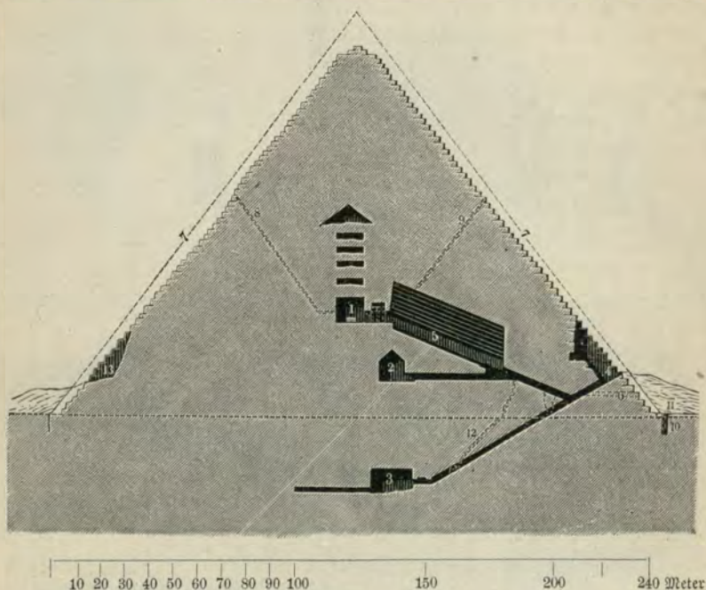
Fig. 24. Das Innere der Großen Pyramide.
