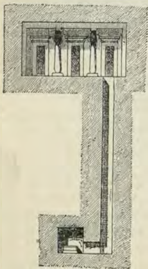
Fig. 26. Oberes Zimmer, Schacht und Grufte.
