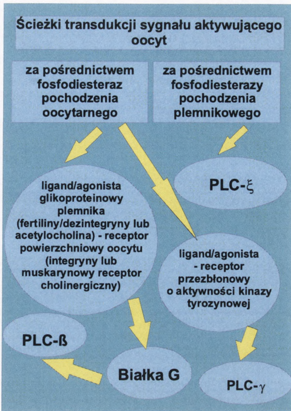
Rys. 2. Scenariusz udziału fosfodiesteraz oocytu i plemnika z podklasy fosfolipaz/fosfoinozytydaz typu C (PLC) w inicjacji przekazywania sygnału aktywującego komórkę jajową (szczegółowe objaśnienia w tekście).
