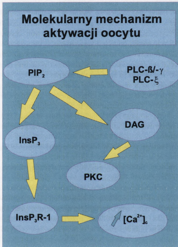
Rys. 3. Schemat szlaków transdukcji sygnału aktywującego w dojrzalym mejotycznie oocycie. Główne ogniwa mechanizmu aktywacji oocytu stanowią: fosfolipazy C podtypu \beta oraz \gamma (PLC- \beta - \gamma ) lub izoforma \xi fosfolipazy C (PLC- \xi ); fosfatydyloinozytolo-4,5-bisfosforan (PIP 2 ); myo -inozytolo-1,4,5-trisfosforan (InsP 3 ); receptory InsP 3 -zależnych kanałów wapniowych (InsP 3 R); kationy wapnia; 1,2-diacylglicerol (DAG) oraz kinaza białkowa C (PKC) (szczegółowe objaśnienia w tekście).
