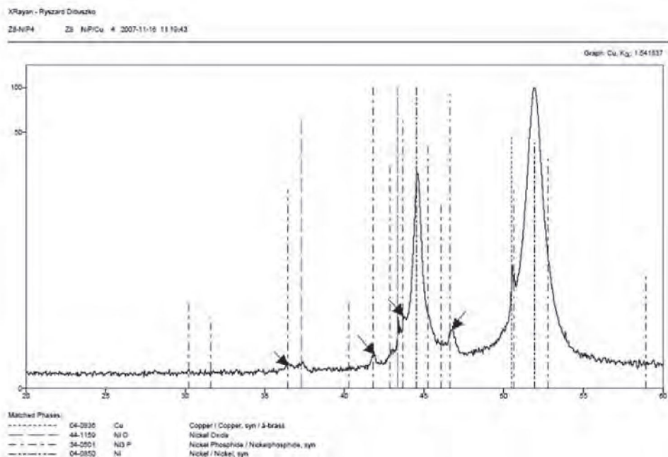
Rys. 2. Dyfraktogram przedstawiający skład stopu Ni-P w powłoce gradientowej z kąpieli C przy gęstości prądu rosnącej skokowo od 5 do 25 A/dm 2 .
