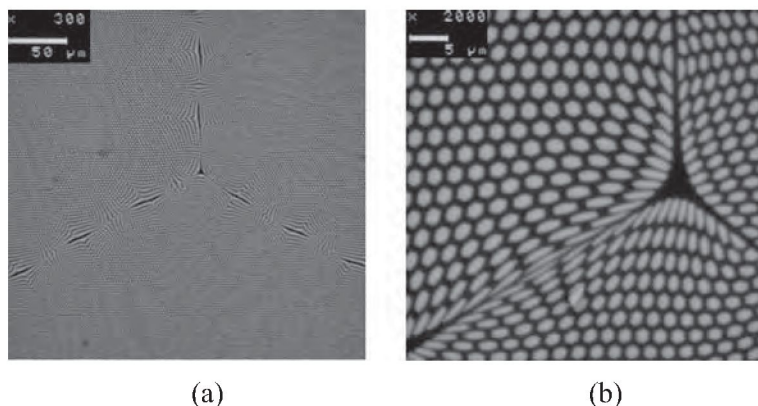
Rys. 22. Deformacje struktury PG-3B o P_{\text{calc}} \approx 3,5 \text{ mm}^2 : (a) poważne defekty powstałe w ostatnim procesie integracji oraz granice elementów pośrednich; (b) zbliżenie 2000x poważnego defektu zaprezentowanego na zdjęciu obok.
