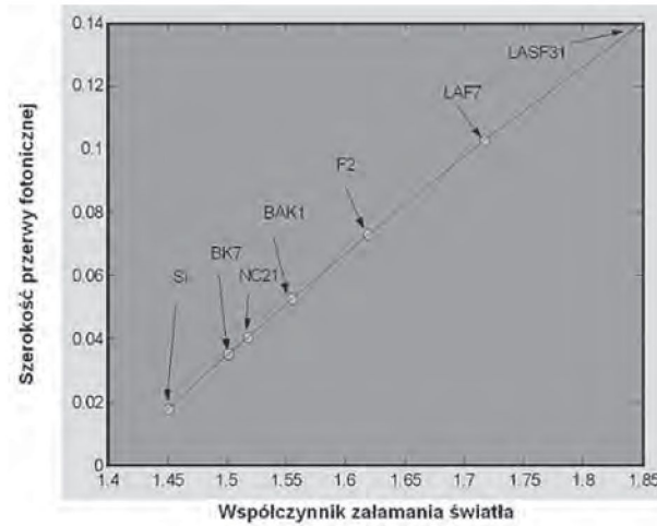
Rys. 1. Szerokość przerwy fotonicznej powietrzno-szklanego kryształu 2-D o heksagonalnej siatce dla kilku wieloskładnikowych szkieł w funkcji wielkości współczynnika załamania światła ( d/A = \text{const} , \lambda = \text{const} ).
