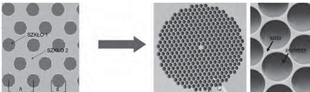
Rys. 3. Periodyczna struktura dwuszkłana jako analogia struktury powietrzno-szkłanej włókna PCF (na zdjęciu po prawej światłowod foniczny wykonany przez US Naval Research Laboratory z zaznaczonymi obszarami szklanymi i powietrznymi).
