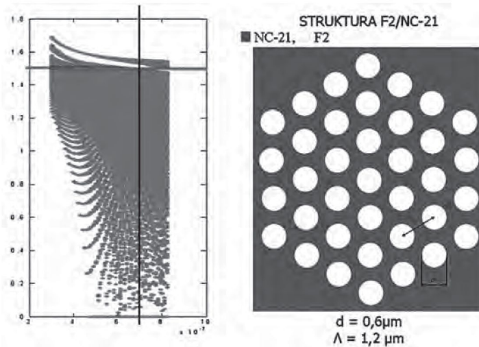
Rys. 12. Pasma wzbronione dla struktury F2/NC-21 o d/\Lambda = 0,5 .
