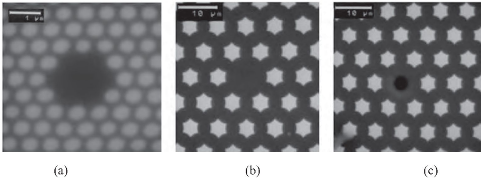
Rys. 7. Periodyczne struktury dwuszklane uzyskanych w ITME włókien PCF-PBG: (a) struktura uzyskana metodą układania pręcików dwuszkłanych; (b) struktura uzyskana metodą układania naprzemiennego dwóch rodzajów pręcików szklanych; (c) struktura powstała z preformy wykonanej z pręcików ułożonych naprzemiennie, z kapilarą w części centralnej [17-20].
