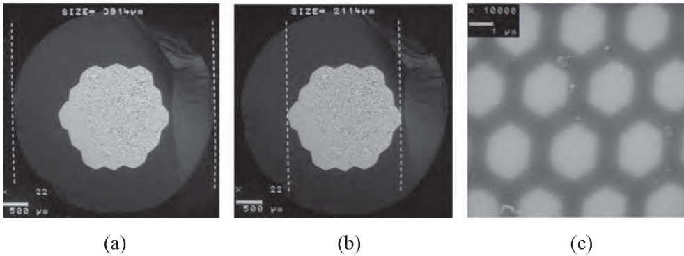
Rys. 20. Zdjęcia SEM struktury PG-3B ( D \approx 2114 \mu\text{m} , P_{\text{calc}} \approx 3,5 \text{ mm}^2 ) umieszczonej w matrycy szklanej o średnicy \sim 4,0 \text{ mm} : (a) powiększenie 22x – widok na strukturę, (b) średnica zaimplementowanej rozległej struktury periodycznej, (c) powiększenie 10000x – inkluzje przyjęły kształt rozciągniętych sześciokątów.
