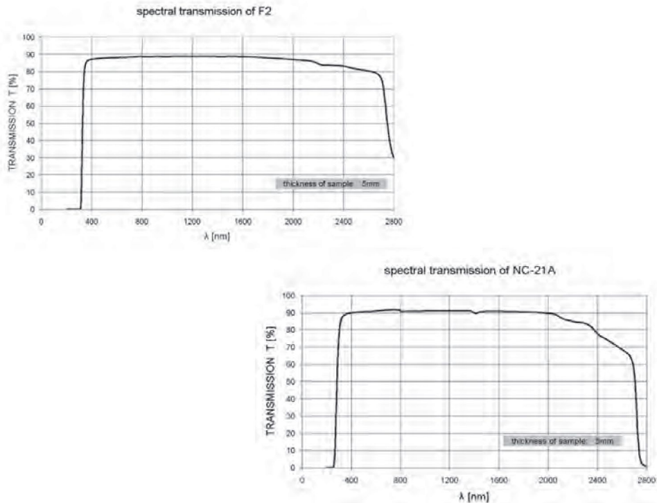
Rys. 9. Widma transmitancji dla szkieł F2 i NC-21
