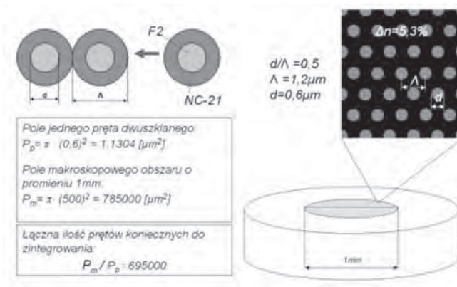
Rys. 8. Oszacowanie ilości niezbędnych do integracji prętów dwuszkłanych dla struktury F2/NC-21 o określonych parametrach d = 0,6 \mu\text{m} i d/\Lambda = 0,5 .
