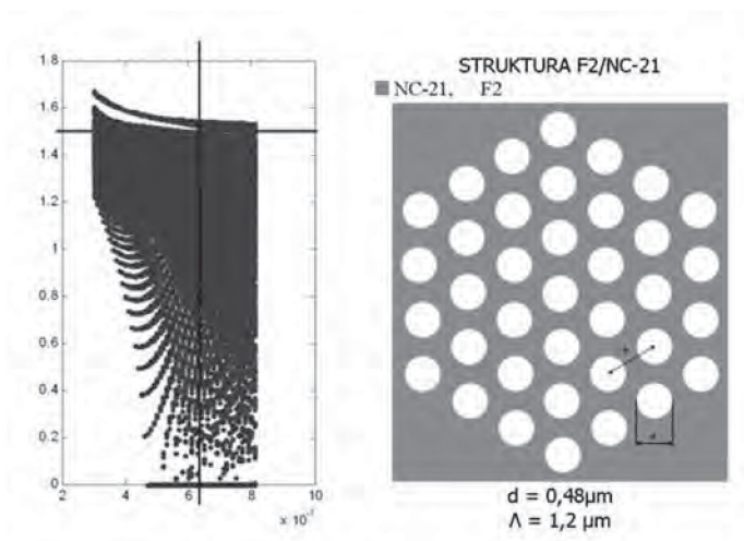
Rys. 13. Pasma wzbronione dla struktury F2/NC-21 o d/\Lambda = 0,4 .
