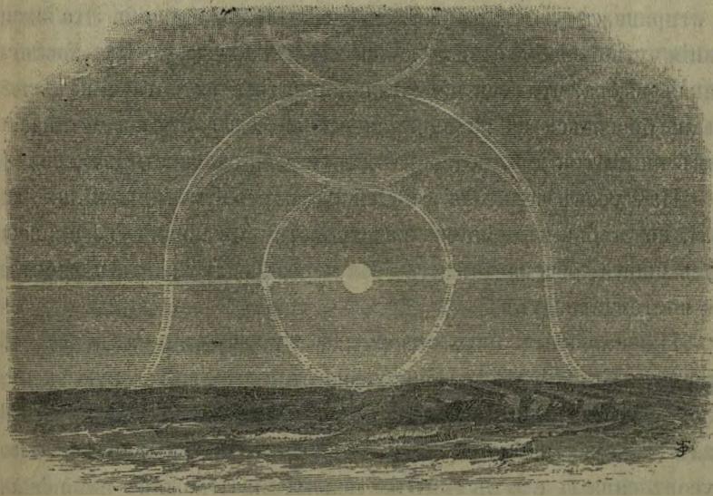
Рефракція.
