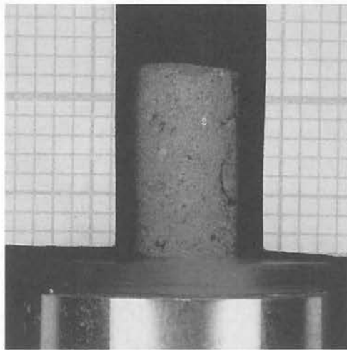
Fig. 4. Mikrordzeń na obrotowym stoliku napędzanym silnikiem krokowym (wstępna wersja).
