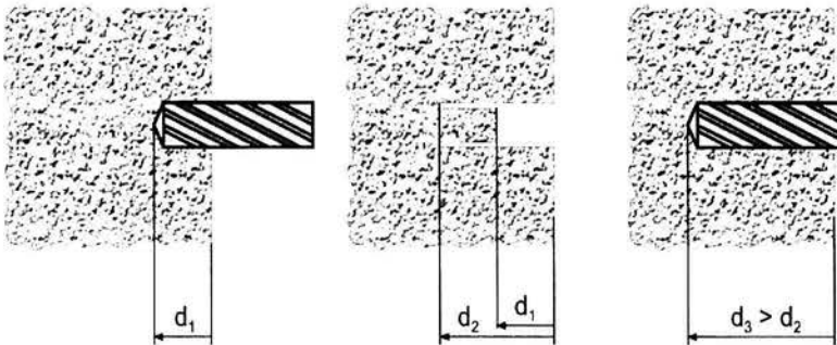
Fig. 3. Core-from-depth procedure.
