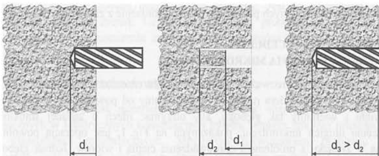
Fig. 3. Sposób pobierania rdzeni z głębi materiału.
