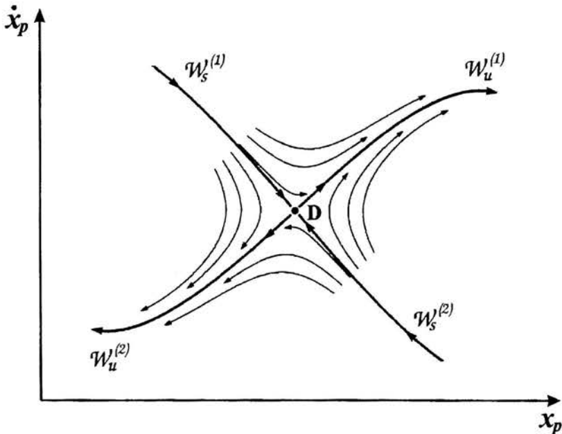
Rys. 6. Przykład niestatecznego rozwiązania T -periodycznego - siodła ; W_s^{(1,2)} , W_u^{(1,2)} reprezentują odpowiednio stateczne i niestateczne rozmaitości siodła D.
