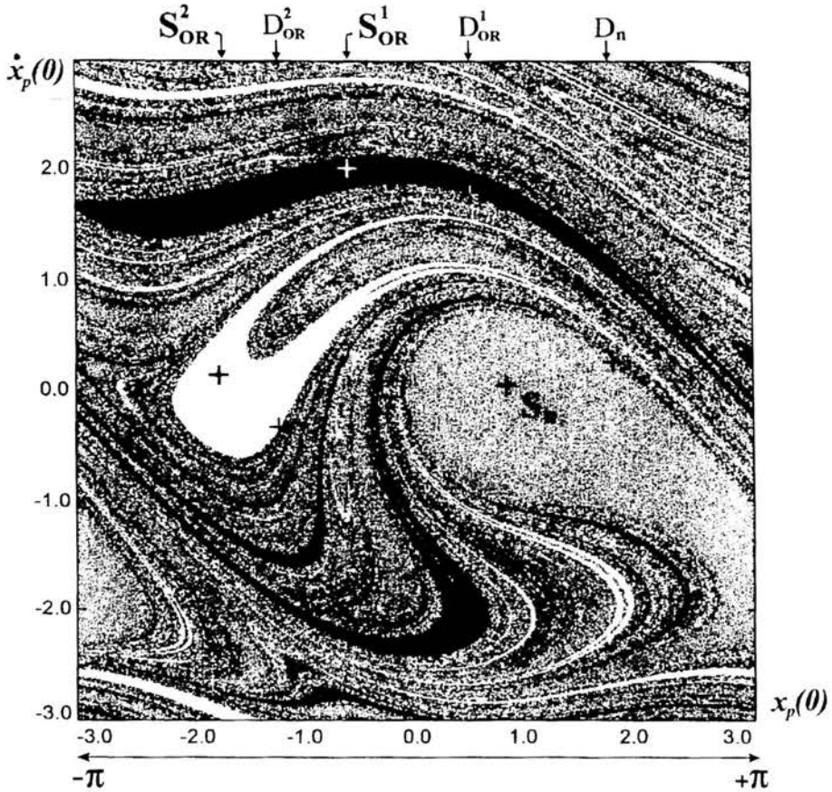
Rys. 13. Obszary przyciągania trzech współistniejących atraktorów (szary - S_n , czarny - S_{OR}^1 , biały - S_{OR}^2 ); F = 0.50 , \omega = 0.58
