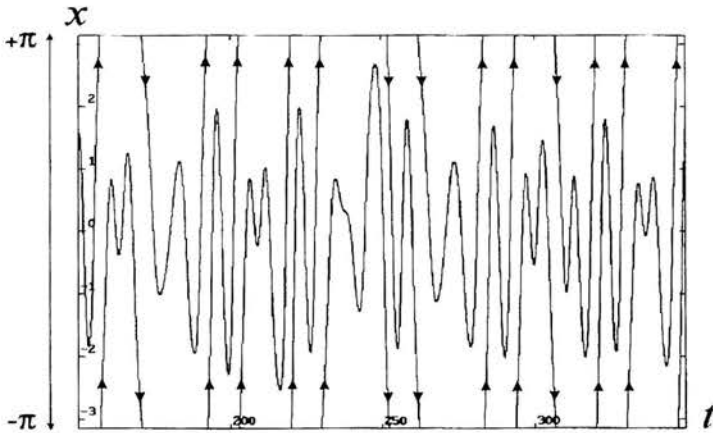
Rys. 16. Przebieg czasowy wychYLENIA przy chaosie trwałym, F = 0.6 , \omega = 0.69 ; strzałki wskazują kierunki obrotów wahadła
