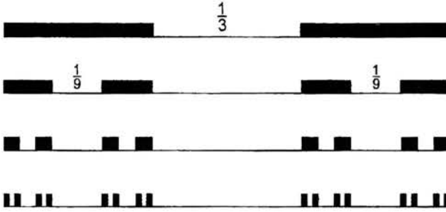
Rys. 19. Cztery pierwsze iteracje zbioru Cantora
