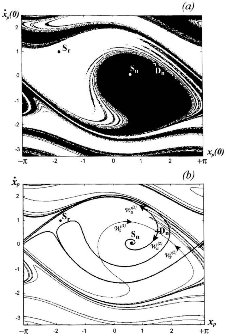
Rys. 11. F = 0.27 , \omega = 0.73 ; (a) obszary przyciągania atraktorów S_n (czarny) i S_r (biały); (b) stateczne (linie cienkie) i niestateczne (linie grube) rozmaitości siodła D_n
