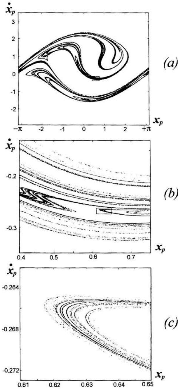
Rys. 17. Mapa Poincarégo atraktora chaotycznego; (a) cały atraktor; (b), (c) - kolejne powiększenia fragmentów atraktora
