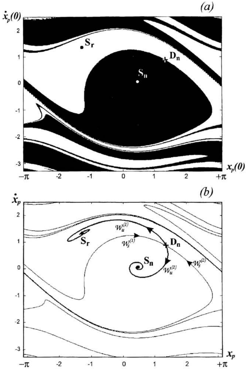
Rys. 10. F = 0.20 , \omega = 0.75 ; (a) obszary przyciągania atraktorów S_n (czarny) i S_r (biały); (b) stateczne (linie cienkie) i niestateczne (linie grube) rozmaitości siodła D_n
