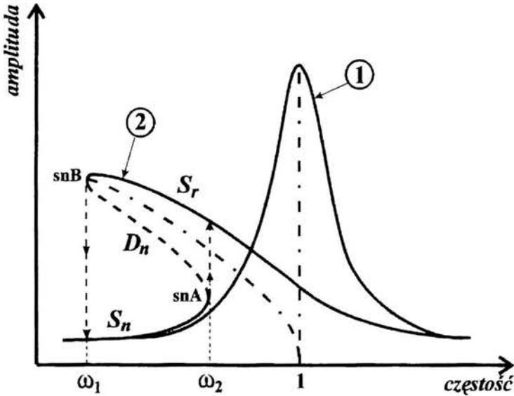
Rys. 2. Krzywe rezonansowe układu liniowego (1) oraz słabo nieliniowego (2)
