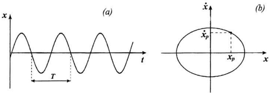
Rys. 3. Graficzna ilustracja ruchu periodycznego; (a) przebieg czasowy, (b) portret fazowy
