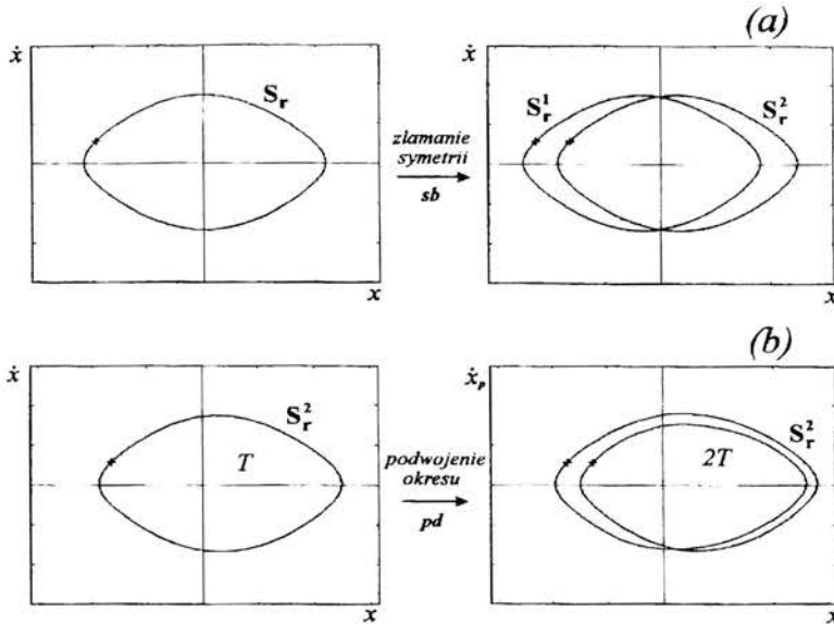
Rys. 9. Ilustracja bifurkacji złamania symetrii (a) oraz bifurkacji podwojenia okresu (b) na płaszczyźnie fazowej
