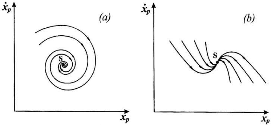
Rys. 5. Przykłady statecznych rozwiązań T -periodycznych - atraktorów ; (a) „ognisko” (b) „węzeł”
