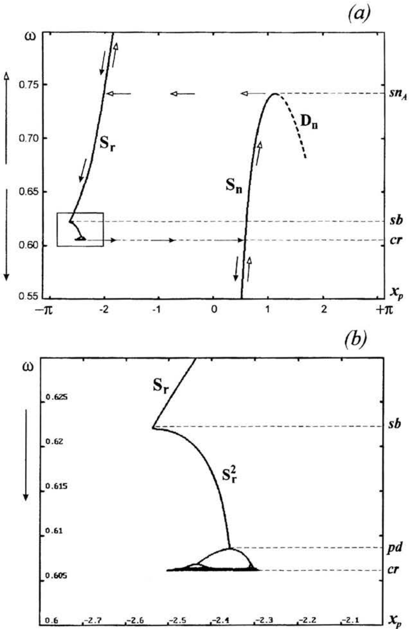
Rys. 8. Wykres bifurkacyjny, F = 0.35 ; (a) przy zmniejszaniu oraz zwiększaniu parametru bifurkacyjnego \omega , (b) powiększony fragment wykresu oznaczony prostokątem na rys. 8a, przy zmniejszaniu parametru \omega
