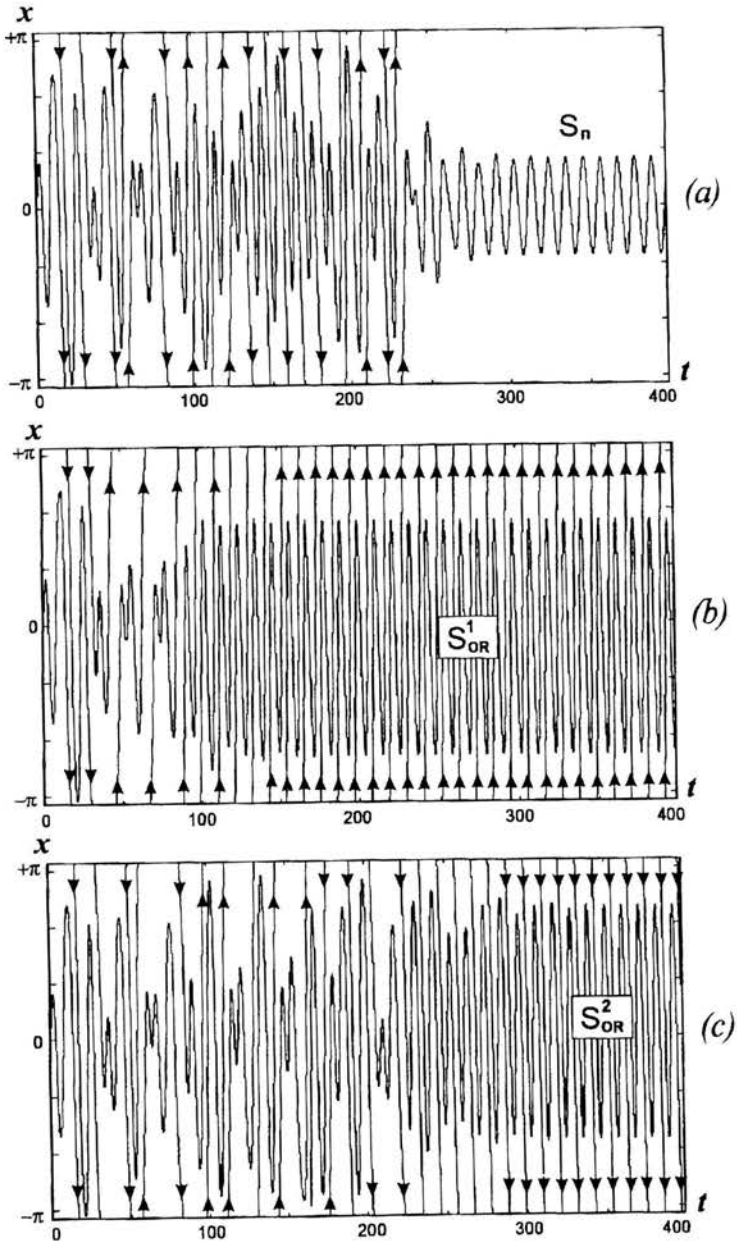
Rys. 14. Trzy przebiegi czasowe ruchu układu przy bardzo bliskich wartościach warunków początkowych, F = 0.50 , \omega = 0.58 (strzałki wskazują kierunki obrotów wahadła); (a) x(0) = -0.220 , \dot{x}(0) = 0.010 , (b) x(0) = -0.218 , \dot{x}(0) = 0.010 , (c) x(0) = -0.220 , \dot{x}(0) = 0.000
