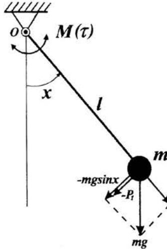
Rys. 1. Model wahadła matematycznego
