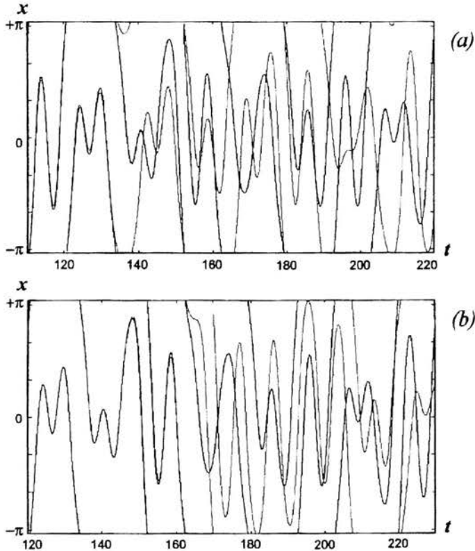
Rys. 18. Ilustracja wrażliwości przebiegu wychyleń w czasie na warunki początkowe: (a) linia czarna - x(0) = 0.606 , \dot{x}(0) = -0.242 , linia szara - x(0) = 0.610 , \dot{x}(0) = -0.242 ; (b) linia czarna - lkc = 100 , linia szara - lkc = 300 ( lkc - liczba kroków na cykl).
