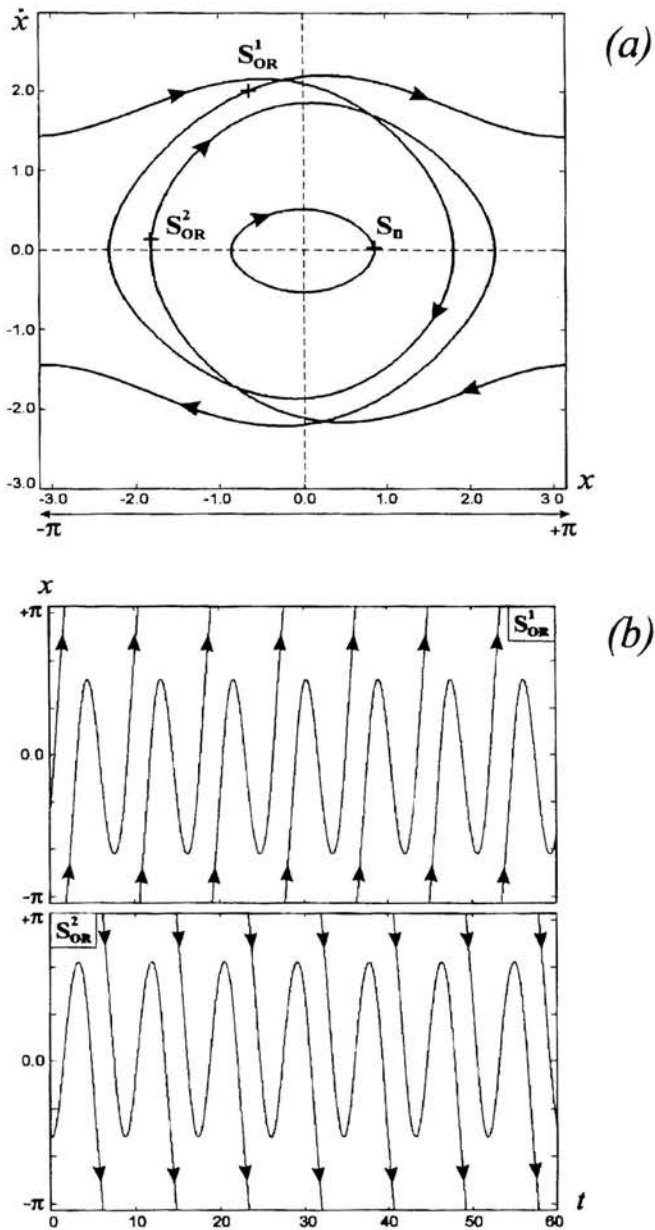
Rys. 12. (a) portrety fazowe trzech współistniejących atraktorów S_n , S_{OR}^1 , S_{OR}^2 przy F = 0.50 , \omega = 0.58 ; (b) przebiegi czasowe atraktorów oscylacyjno-rotacyjnych S_{OR}^1 , S_{OR}^2 .
