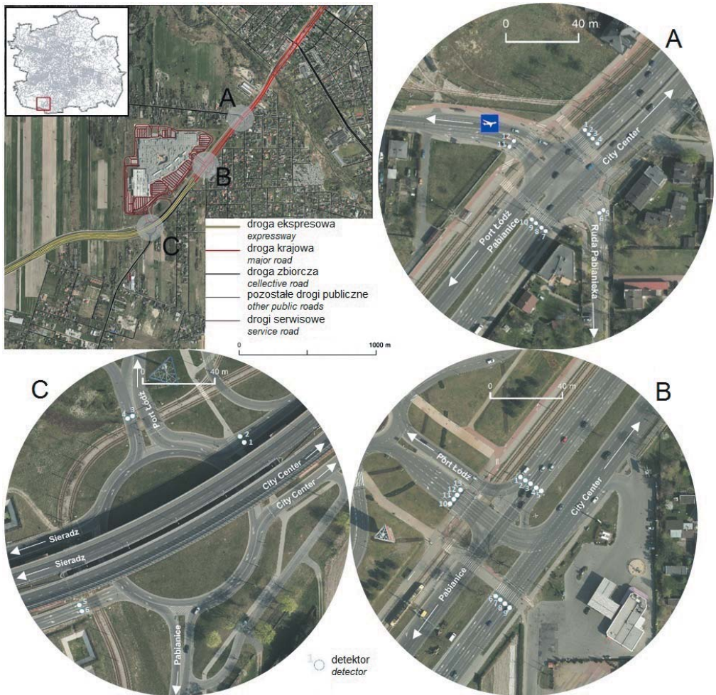
Ryc. 1. Rozmieszczenie detektorów (pętli indukcyjnych) na drogach w rejonie Portu Łódź Location of detectors (inductive loops) on roads near Port Łódź
