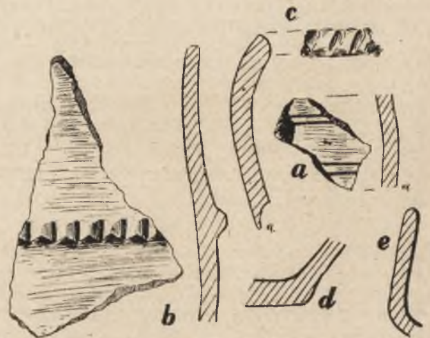
Ryc. 6. Wiankowo, pow. głogowski; miejsce D. Ułamki ceramiki kultury lużyckiej; \frac{1}{2} w. n.
