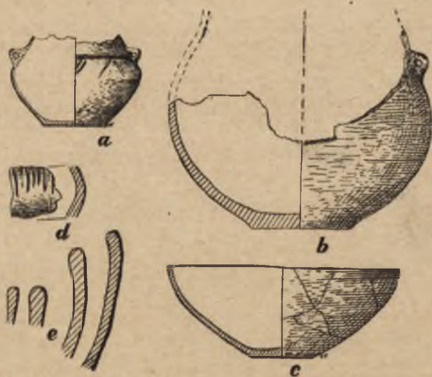
Ryc. 4. Wiąnkowo, pow. głogowski; miejsce B. Zabytki kultury łużyckiej; a) \frac{1}{8} w. n.; b, c) \frac{1}{4} w. n.; d, e) \frac{1}{2} w. n.
