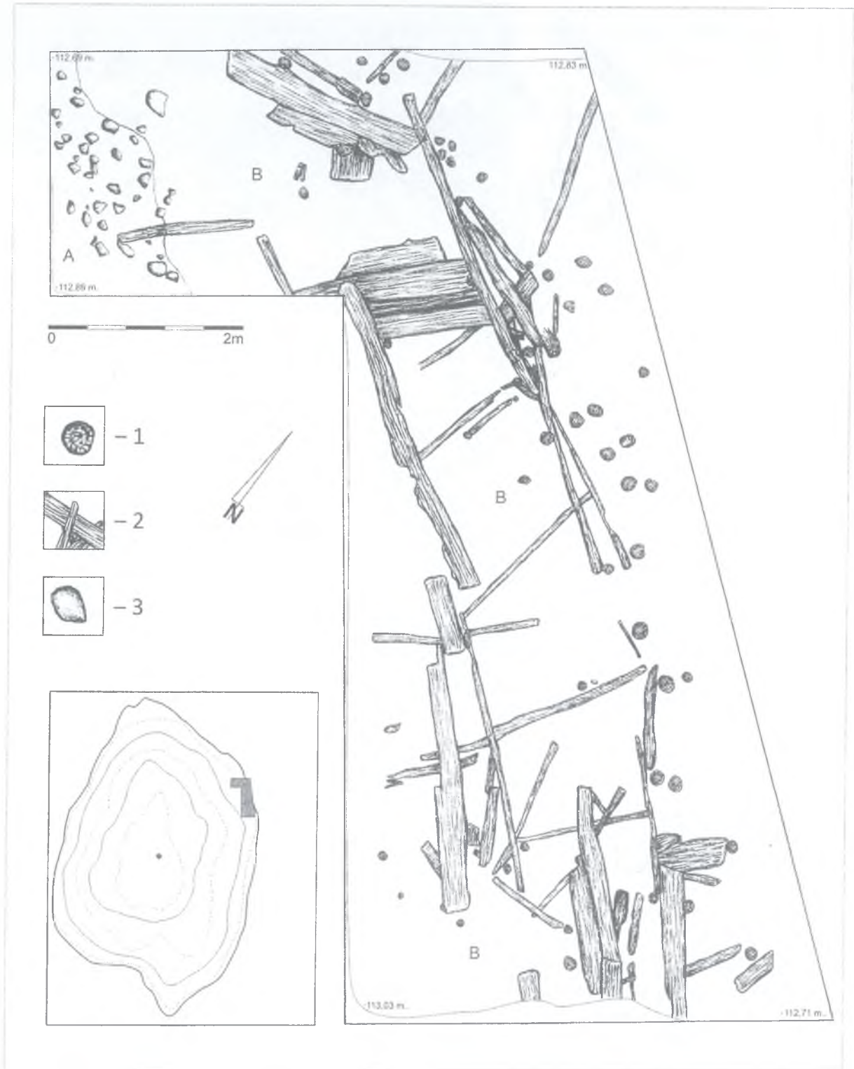
Ryc. 13. Żółte, woj. zachodniopomorskie, stanowisko 33. Wykop 13/06. Rzut poziomy relikwów konstrukcji drewnianych występujących w strefie brzegowej wyspy. 1 – pale; 2 – drewniane elementy konstrukcji nabrzeża; 3 – kamienie; A – drobnoziarnisty piasek; B – osady biogeniczne (rys. B. Kowalewska)
