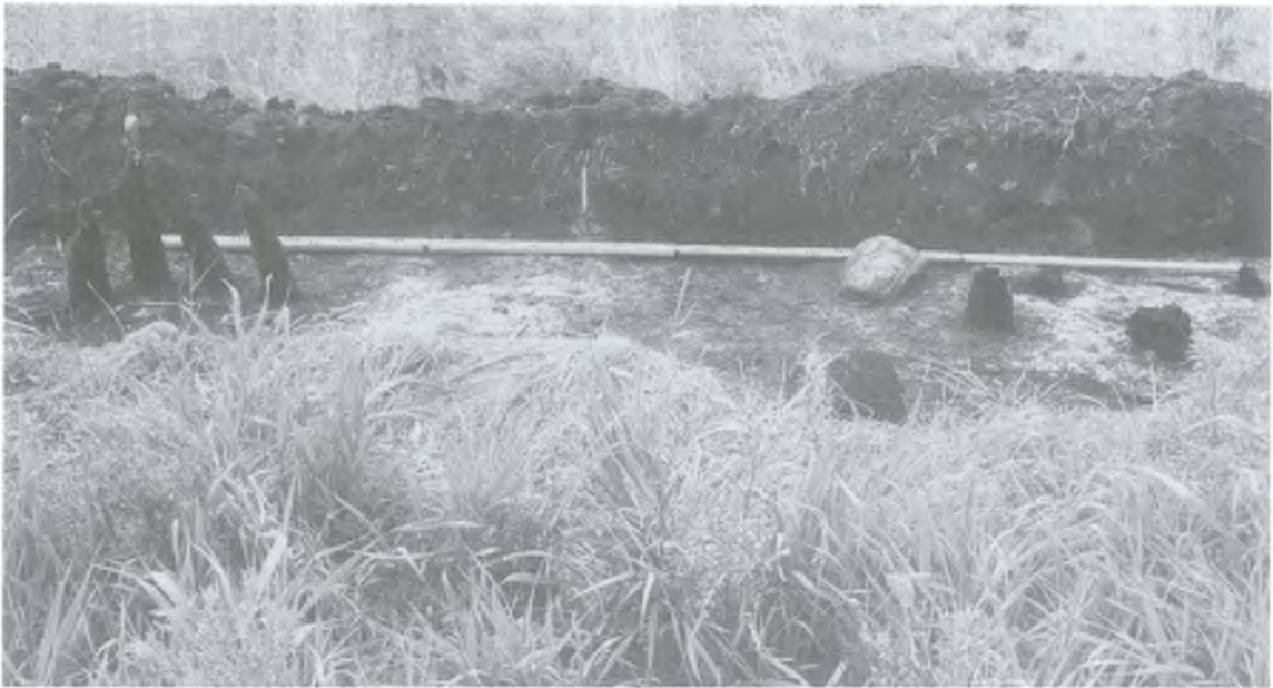
Ryc. 14. Parsęcko, woj. zachodniopomorskie, stanowisko 2. Wiązki pali konstrukcyjnych mostu prowadzącego na wyspę (widok od północy, fot. R. Kaźmierczak)
