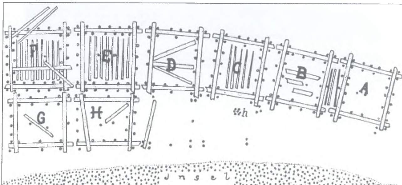
Ryc. 3. Parsęcko, woj. zachodniopomorskie, stanowisko 2. Planigrafia relikwów zabudowy odsłoniętych w latach 60-tych XIX wieku w północnej części wyspy (wg Kasiski 1869)
