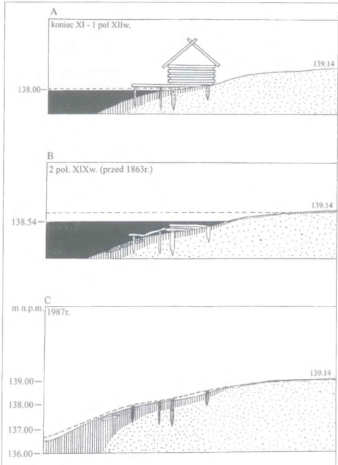
Ryc. 7. Parsęcko, woj. zachodniopomorskie, stanowisko 2. Schemat rekonstrukcji zmian średniego poziomu lustra wody w jeziorze w powiązaniu z rekonstrukcją dookólnej zabudowy (A) oraz jej relikdami (B-C) (wg Gackowski, Jabłoński 1988, ryc. 2)
