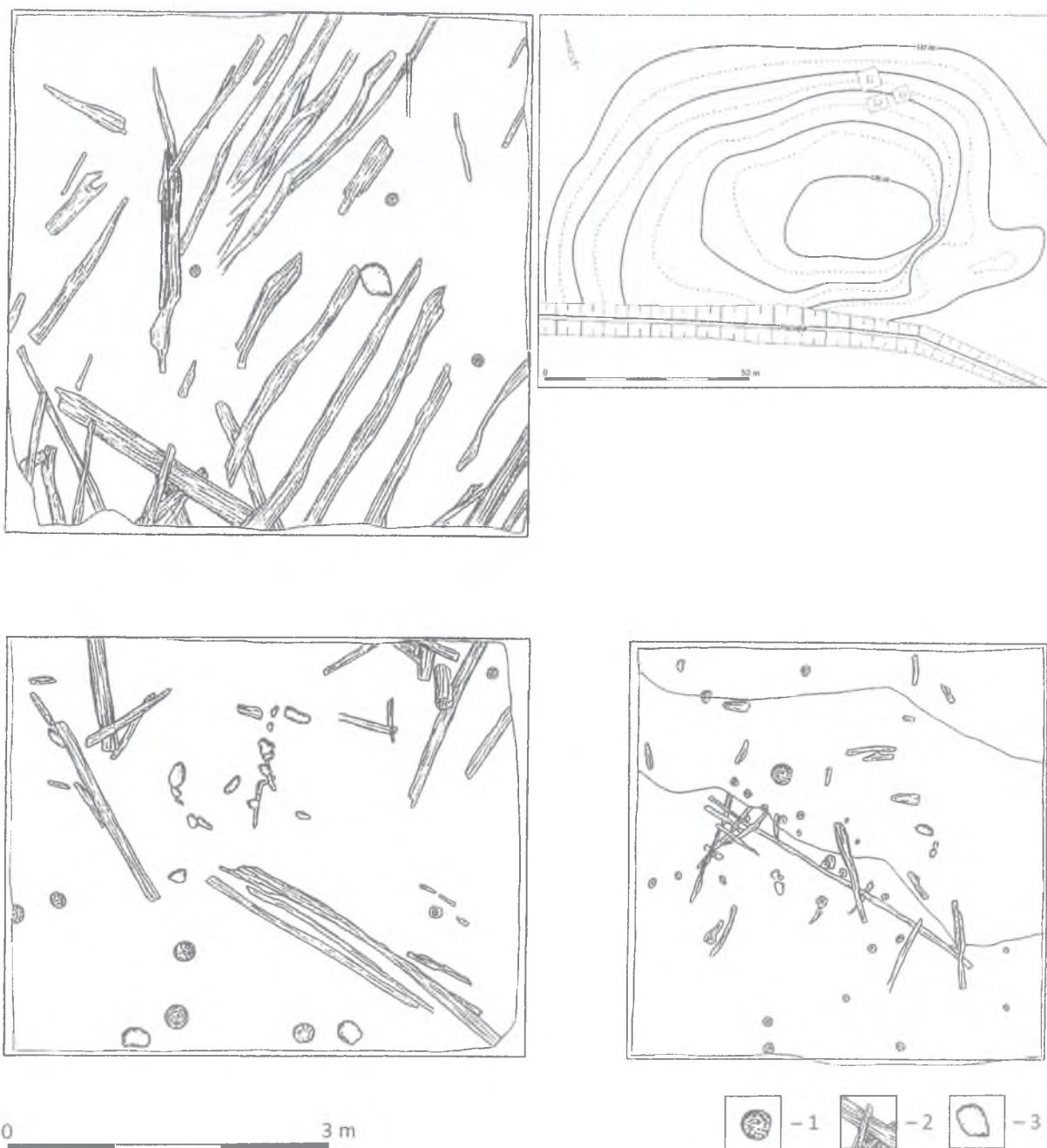
Ryc. 6. Parsęcko, woj. zachodniopomorskie, stanowisko 2. Rzut relikwów konstrukcji drewnianych odsłoniętych w północnej części wyspy w latach 1987-1988. 1 – pale; 2 – elementy poziomych konstrukcji drewnianych; 3 – kamienie (wg Gackowski 1988)
