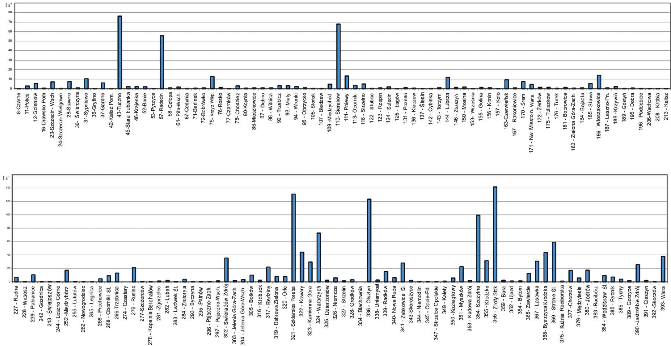
Ryc. 5. Wydajność wypływów wód podziemnych w obrębie arkuszy (numeracja zgodna z zamieszczoną na rycinie 1) Discharge of underground waters within the area covered by the map sheets
