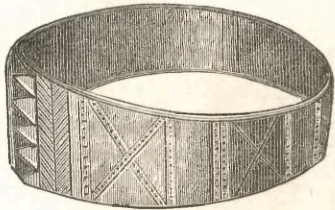
868. \frac{2}{3} .
