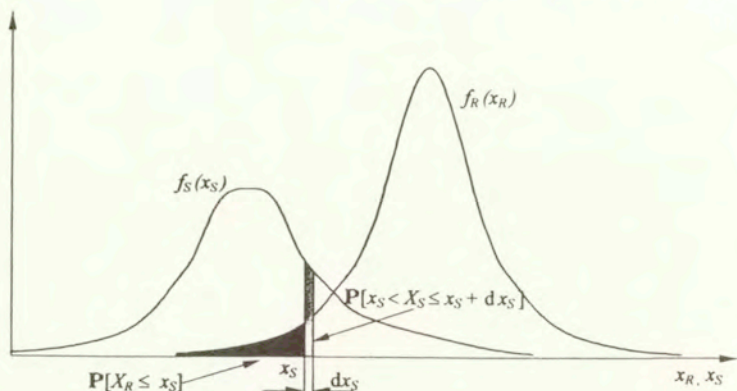
Rys. 2.2: Graficzna reprezentacja całki (2.2b)
