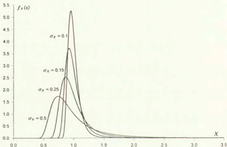
Rys. C.3: Rozkłady Frecheta dla X^0 = 1
