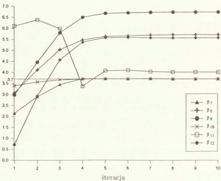
Rys. 4.14: Podejście standardowe. Wskaźniki \beta odpowiadające ograniczeniom 7-12
