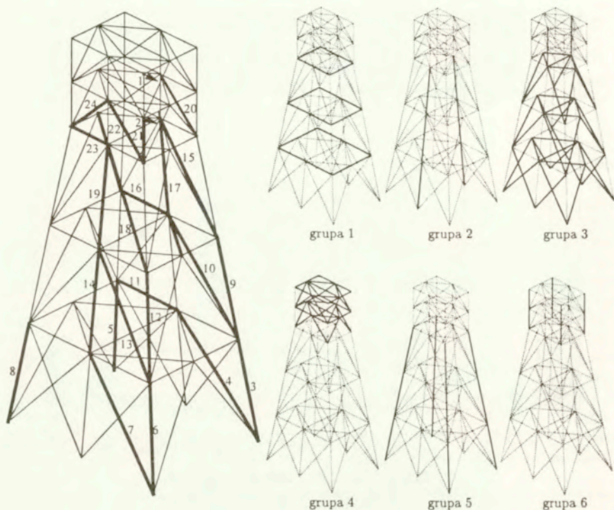
Rys. 4.6: Konstrukcja wsporcza platformy wiertniczej, 1, 2 - warunki przemieszczeniowe, 3-24 - warunki naprężeniowe; grupy elementów
