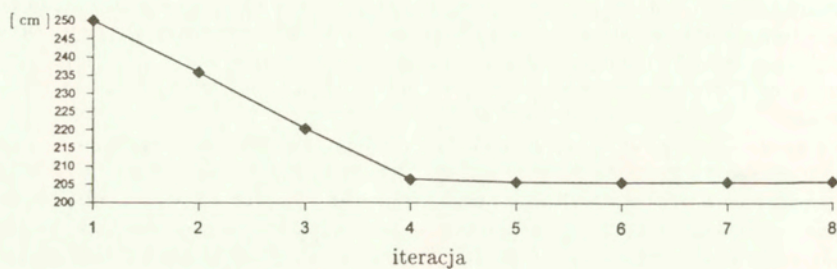
Rys. 5.7: Kopuła kratowa: odległość w planie węzła 1 od węzłów 2-7
