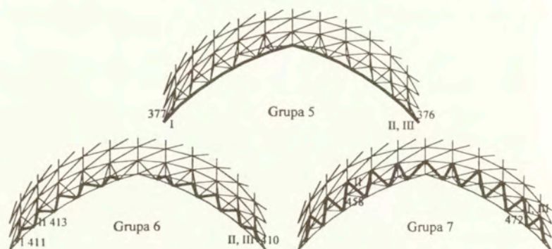
Rys. 3.7: Grupy elementów 5-7; zaznaczono pręty z ograniczeniami naprężeniowymi
