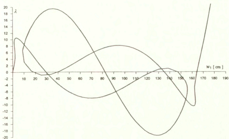
Rys. 5.9: Kopuła kratowa: podstawowa ścieżka równowagi konstrukcji optymalnej
