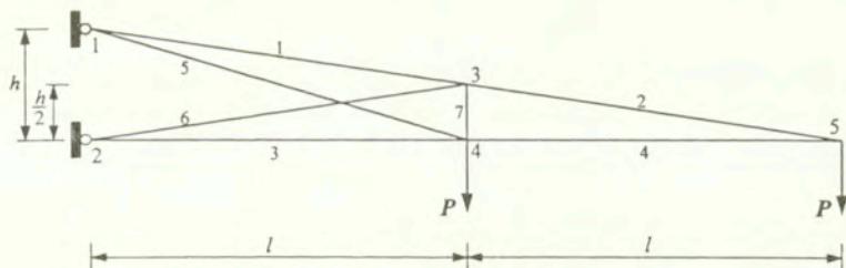
Rys. 2.5: Wspornik kratowy
