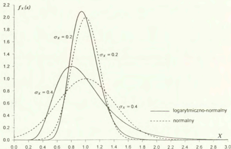
Rys. C.1: Rozkłady normalne i logarytmiczno-normalne dla X^0 = 1
