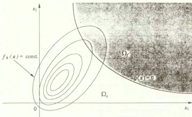
Rys. 2.4: Powierzchnia graniczna g(\mathbf{x}) = 0 , obszar bezpieczny i obszar awarii w przestrzeni zmiennych \mathbf{X}
