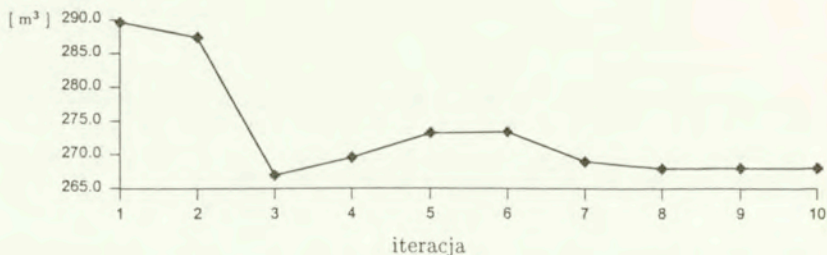
Rys. 4.9: Objętość materiału konstrukcji
