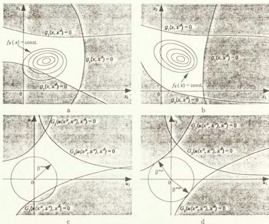
Rys. 3.2: Zadanie optymalizacji niezawodnościowej; przestrzeń \mathcal{X} : a - projekt początkowy, b - projekt optymalny; przestrzeń \mathcal{U} : c - projekt początkowy, d - projekt optymalny
