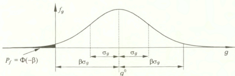
Rys. 2.3: Graficzna interpretacja wzoru (2.5)
