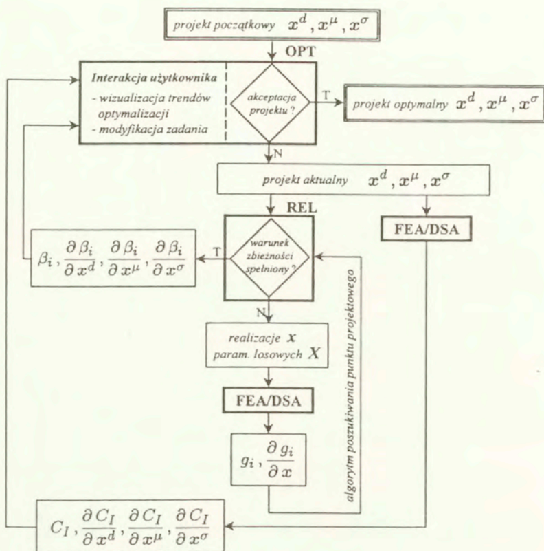
Rys. 3.3: Schemat systemu optymalizacji niezawodnościowej - OPTIREL
