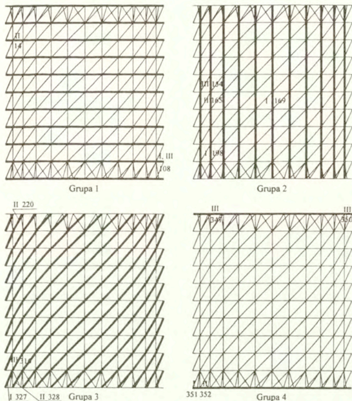
Rys. 3.6: Grupy elementów 1-4; zaznaczono pręty z ograniczeniami naprężeniowymi
