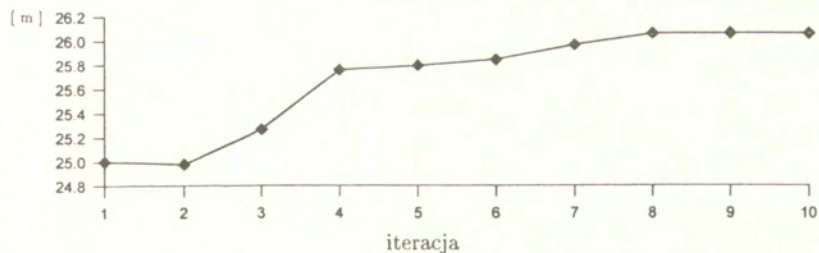
Rys. 4.10: Parametr kształtu - położenie pierwszego pokładu
