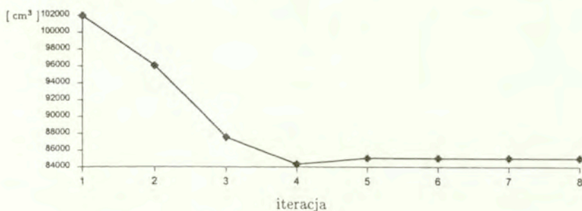
Rys. 5.5: Kopuła kratowa: objętość materiału konstrukcji
