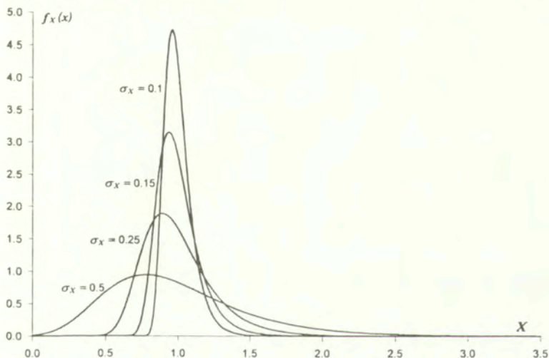
Rys. C.2: Rozkłady Gumbela dla X^0 = 1
