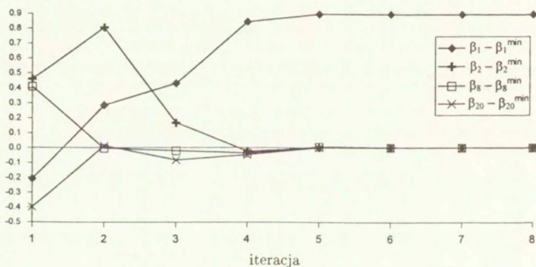
Rys. 5.8: Kopuła kratowa: wartości wybranych ograniczeń niezawodnościowych
