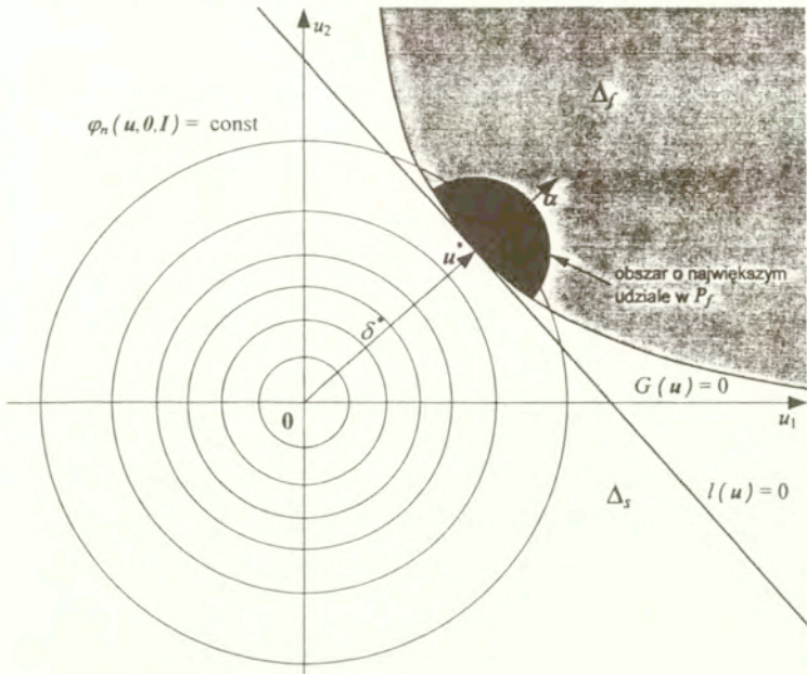
Rys. 2.9: Przybliżenie pierwszego rzędu
