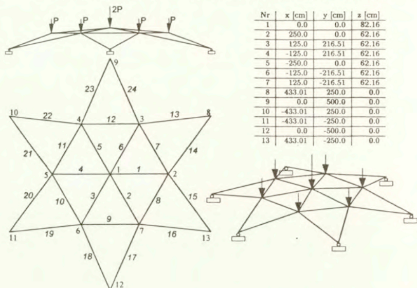
Rys. 5.2: Kopuła kratowa: geometria i obciążenie ( P=20 kN)
