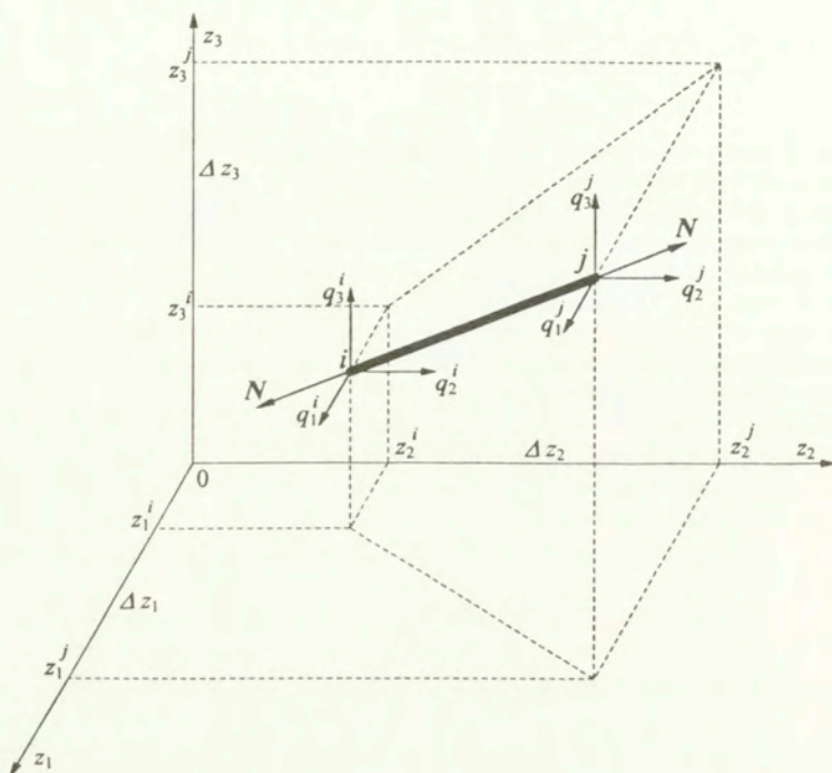
Rys. B.1: Element skończony kratownicy przestrzennej
