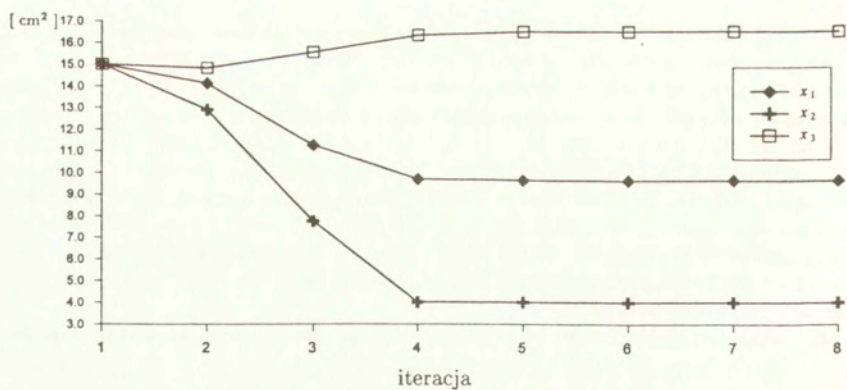
Rys. 5.6: Kopuła kratowa: pola przekrojów grup elementów
