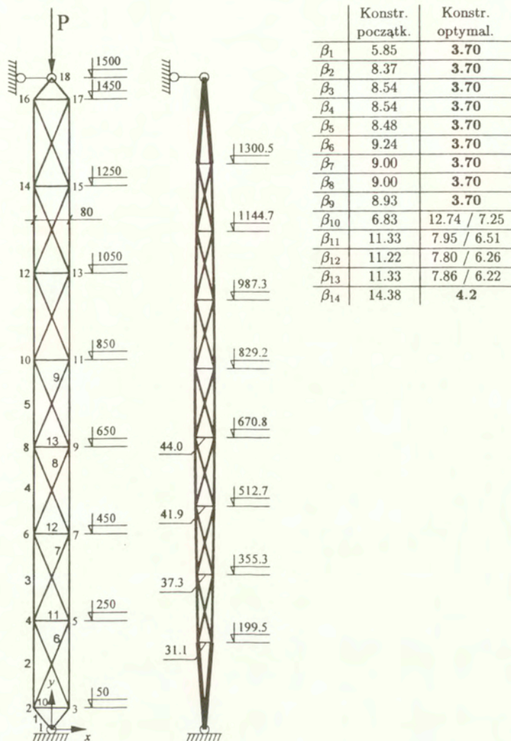
Rys. 5.11: Kolumna kratowa: konfiguracja początkowa i optymalna oraz wartości wskaźników niezawodności
