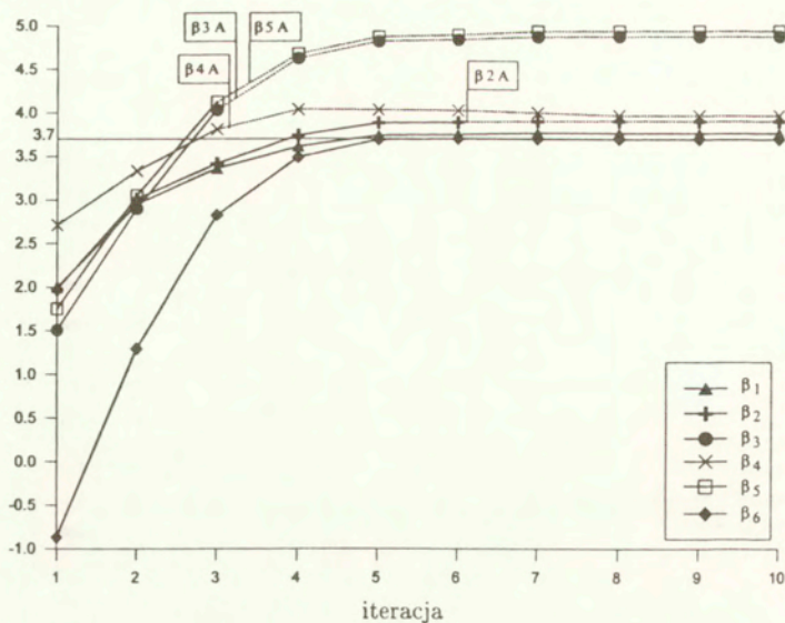
Rys. 4.17: Optymalizacja interaktywna. Wskaźniki \beta odpowiadające ograniczeniom 1-6
