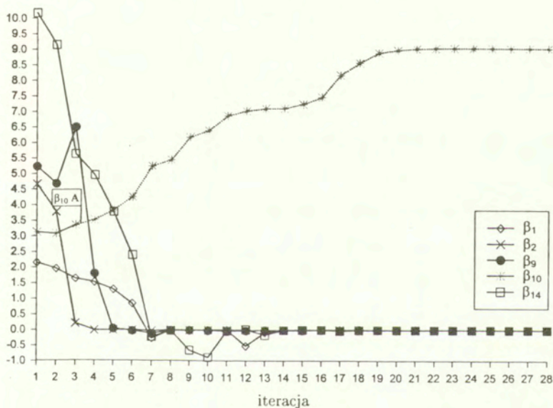
Rys. 5.13: Słup kratowy: wartości wybranych ograniczeń niezawodnościowych
