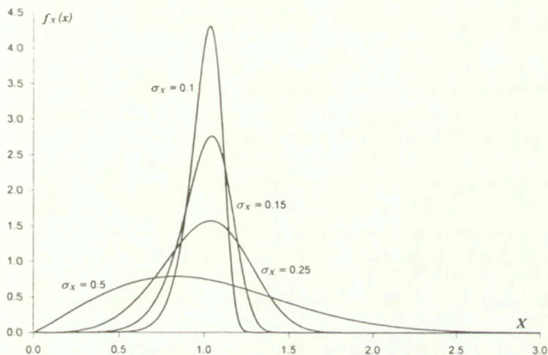
Rys. C.4: Rozkłady Weibulla dla X^0 = 1 i \epsilon = 0
