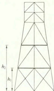
Rys. 4.8: Parametry kształtu - położenie dwóch dolnych pokładów
