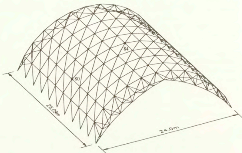
Rys. 3.4: 474-elementowa kratownica przestrzenna w kształcie powłoki cylindrycznej
