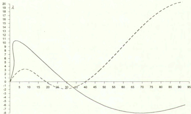
Rys. 5.10: Kopuła kratowa: linia przerywana - ścieżka równowagi konstrukcji początkowej, linia ciągła - ścieżka równowagi konstrukcji optymalnej
