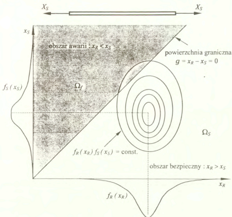
Rys. 2.1: Problem niezawodności pręta rozciąganego
