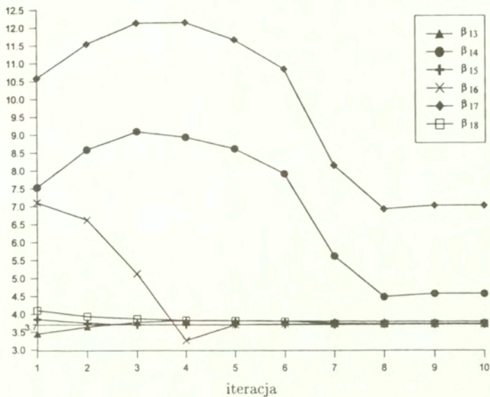
Rys. 4.15: Podejście standardowe. Wskaźniki \beta odpowiadające ograniczeniom 13-18
