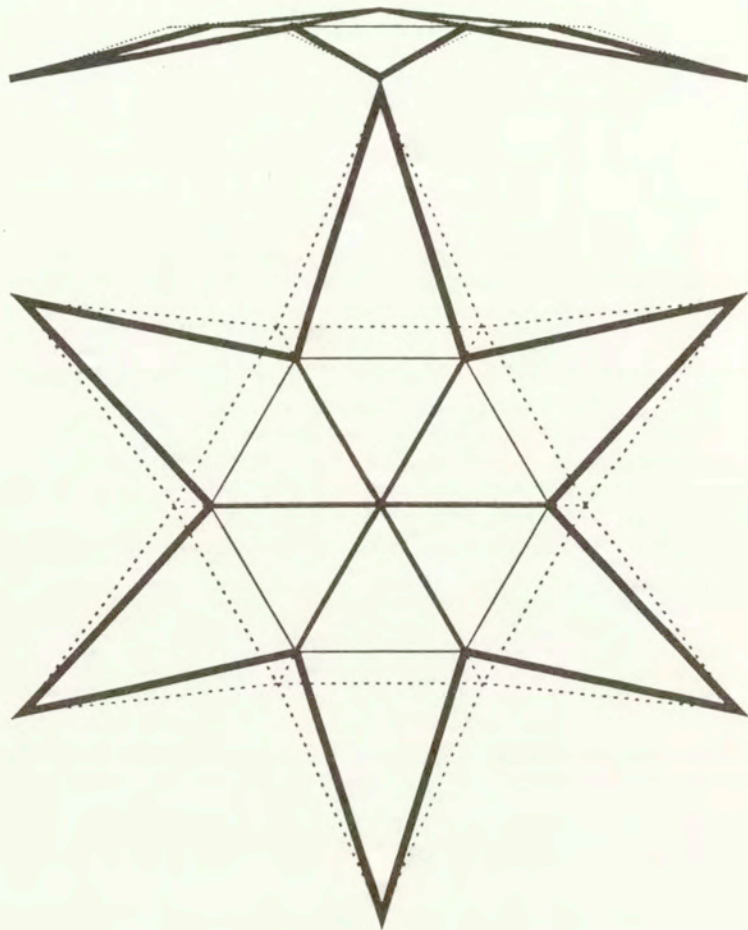
Rys. 5.4: Kopuła kratowa: konfiguracja optymalna
