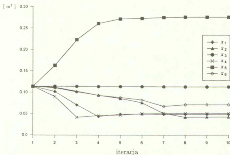
Rys. 4.12: Pola przekrojów grup elementów
