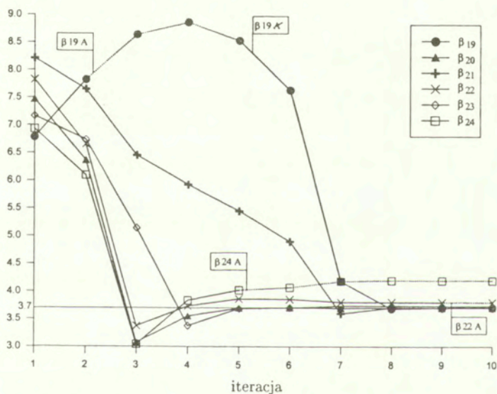
Rys. 4.20: Optymalizacja interaktywna. Wskaźniki \beta odpowiadające ograniczeniom 19-24
