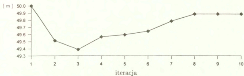
Rys. 4.11: Parametr kształtu - położenie drugiego pokładu
