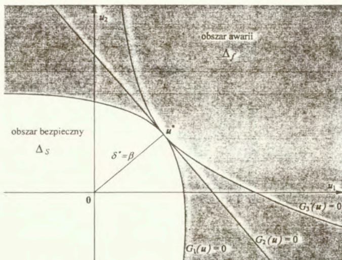
Rys. 2.7: \beta - wskaźnik niezawodności Hasofera-Linda, \mathbf{u}^* - punkt projektowy
