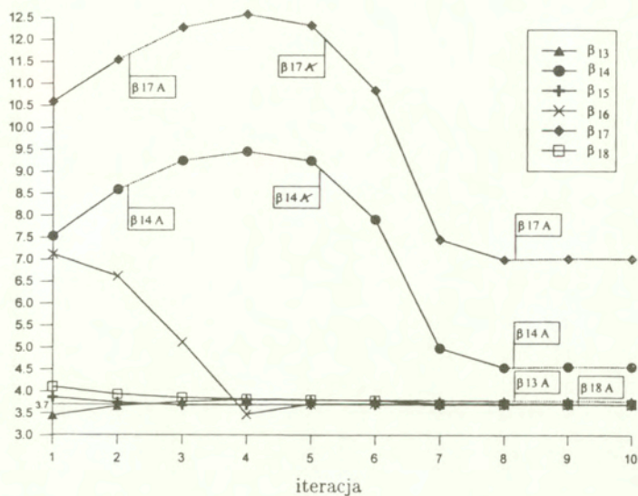
Rys. 4.19: Optymalizacja interaktywna. Wskaźniki \beta odpowiadające ograniczeniom 13-18
