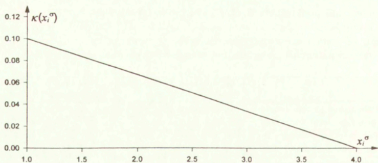
Rys. 3.11: Funkcja \kappa(x_i^\sigma)
