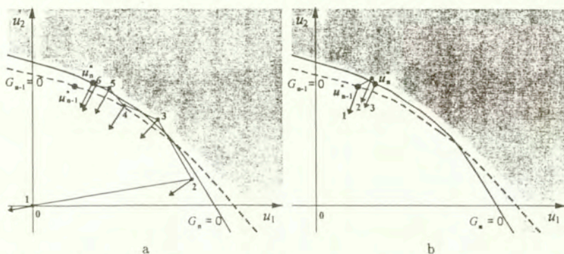
Rys. 4.1: a - algorytm poszukiwania punktu projektowego startuje z punktu \mathbf{u} = 0 b - metoda PPP, algorytm startuje z poprzedniego punktu projektowego, \mathbf{u}_{n-1}^*
