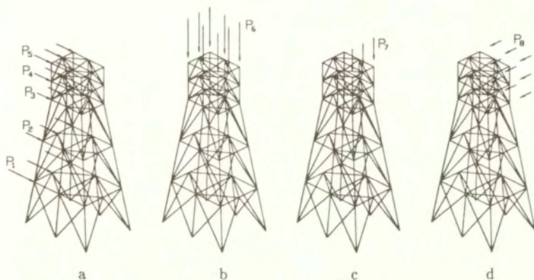
Rys. 4.7: Schematy obciążenia
