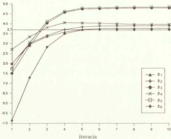
Rys. 4.13: Podejście standardowe. Wskaźniki \beta odpowiadające ograniczeniom 1-6
