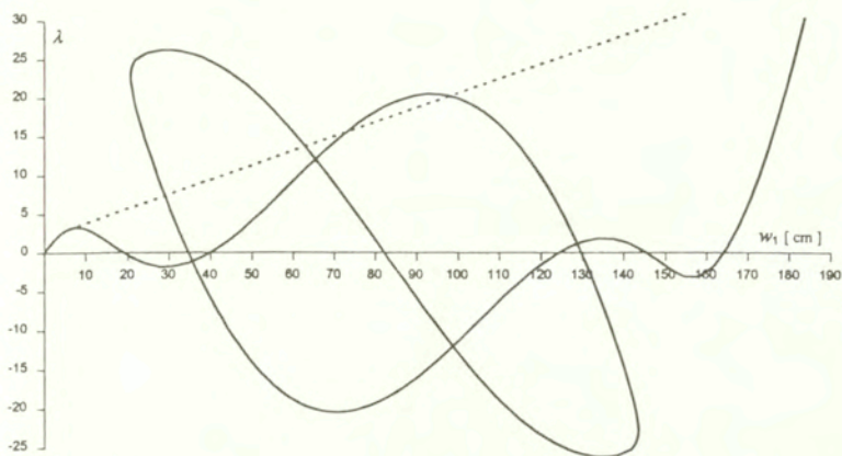
Rys. 5.3: Kopuła kratowa: linia ciągła - podstawowa ścieżka równowagi, linia przerywana - uproszczona ścieżka równowagi pokrytycznej
