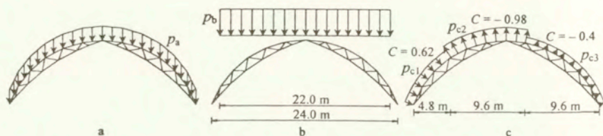
Rys. 3.8: Podstawowe schematy obciążenia: a - obciążenie stałe, b - obciążenie śniegiem, c - obciążenie wiatrem
