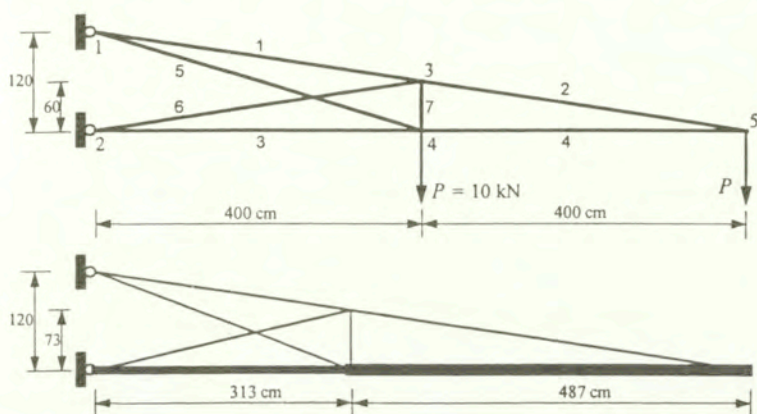
Rys. 3.9: Wsparnik kratowy, optymalizacja kosztu początkowego: u góry - konstrukcja początkowa, u dołu - konstrukcja optymalna
