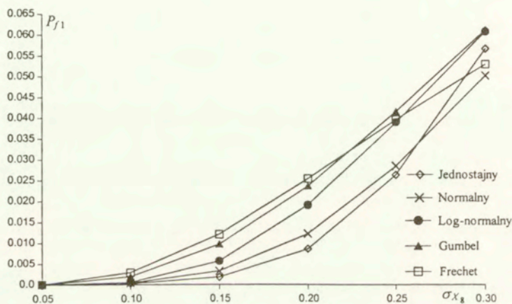
Rys. 2.11: Prawdopodobieństwo awarii dla różnych rozkładów prawdopodobieństwa oraz wartości odchylenia standardowego mnożnika obciążenia
