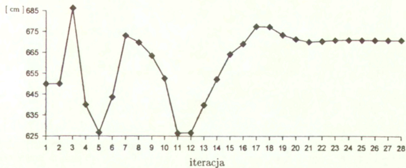
Rys. 5.14: Słup kratowy: położenie poziomego stężenia 8-9
