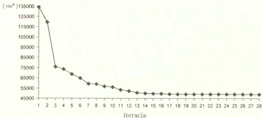
Rys. 5.12: Słup kratowy: objętość materiału konstrukcji
