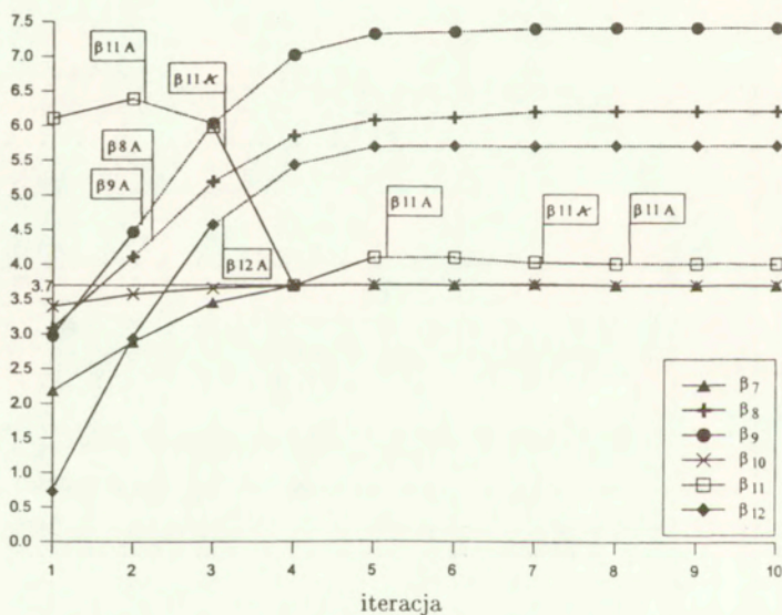
Rys. 4.18: Optymalizacja interaktywna. Wskaźniki \beta odpowiadające ograniczeniom 7-12
