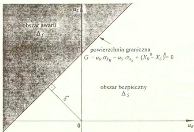
Rys. 2.6: Interpretacja geometryczna wskaźnika niezawodności (2.5)
