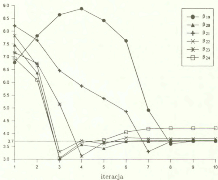
Rys. 4.16: Podejście standardowe. Wskaźniki \beta odpowiadające ograniczeniom 19-24
