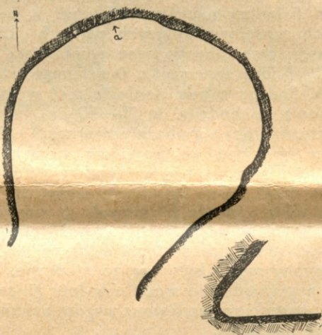
Ryc. 4. Gródek, pow. rówieński. Rzut poziomy i przekrój pionowy (w punkcie a) dolnej części pieca. \frac{1}{30} w. n. — Fig. 4. Gródek, distr. Równe (Volhynie). Plan et coupe transversale de la partie inférieure d'un four ( \frac{1}{30} gr. nat.).
