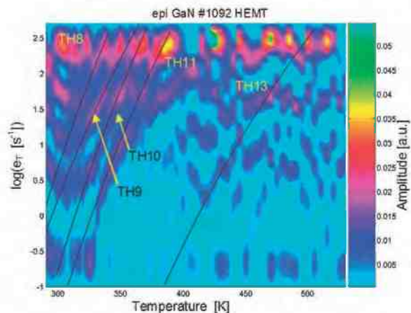
Rys. 17. Obraz prążków widmowych otrzymany za pomocą odwrotnej transformacji Laplace'a dla centrów defektowych wykrytych w niedomieszkowanej warstwie GaN dla tranzystora HEMT, powstały na podstawie relaksacyjnych przebiegów fotoprądu zmierzonych w zakresie temperatur 290 - 530 K.
