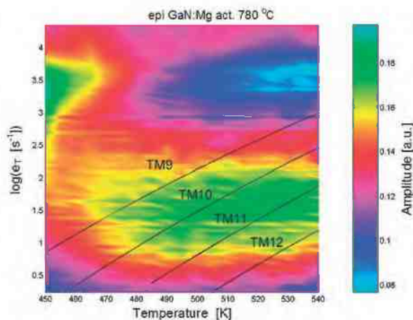
Rys. 9. Obraz korelacyjnych prążków widmowych dla centrów defektowych wykrytych w warstwie GaN:Mg poddanej obróbce termicznej otrzymany na podstawie relaksacyjnych przebiegów fotoprądu zmierzonych w zakresie temperatur 450 - 540 K.
