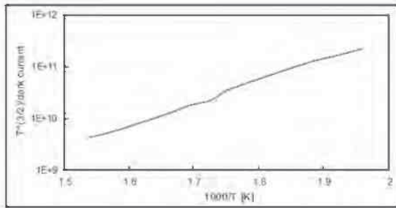
Rys. 13. Wykres prądu ciemnego w funkcji temperatury dla niedomieszkowanej warstwy GaN dla tranzystora HEMT. Wyznaczona energia aktywacji przewodnictwa wynosi 0,85 eV.
