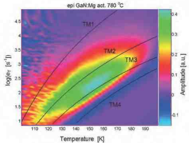
Rys. 5. Obraz korelacyjnych prążków widmowych dla centrów defektowych wykrytych w warstwie GaN:Mg poddanej obróbce termicznej otrzymany na podstawie relaksacyjnych przebiegów fotoprądu zmierzonych w zakresie temperatur 100-200 K.
