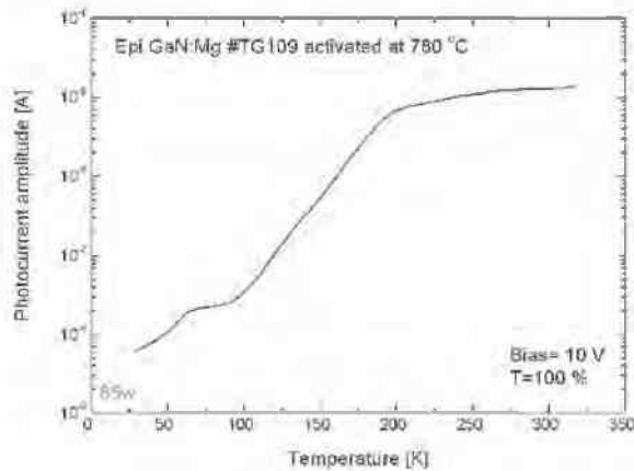
Rys. 4. Temperaturowa zależność amplitudy impulsu fotoprądu w zakresie temperatur 30 - 320 K dla warstwy GaN:Mg poddanej obróbce termicznej w temperaturze 780°C. Strumień fotonów \Phi = 3,13 \times 10^{18} \text{ s}^{-1}\text{cm}^{-2} .
