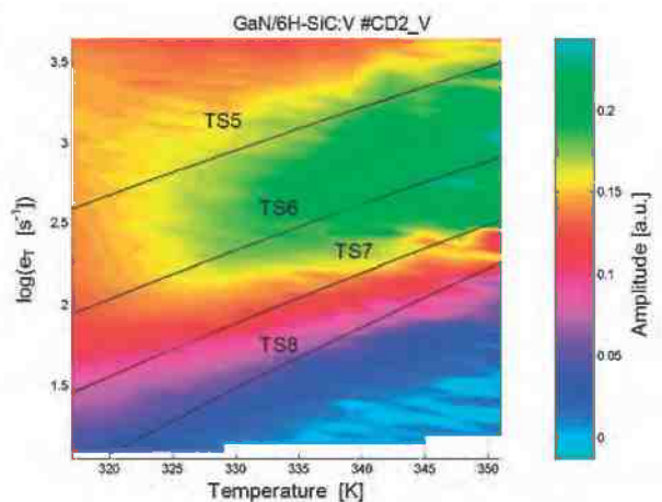
Rys. 25. Obraz korelacyjnych prążków widmowych dla centrów defektowych wykrytych w niedomieszkowanej warstwie GaN osadzonej na podłożu SI 6H-SiC:V otrzymany na podstawie relaksacyjnych przebiegów fotoprądu zmierzonych w zakresie temperatur 315-350 K.
