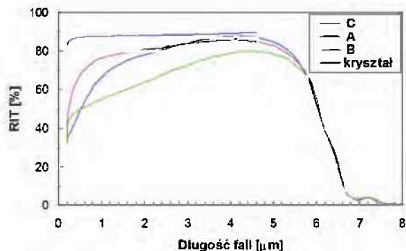
Rys. 6. Zmierzone widmo transmisji RIT dla ceramiki o grubości 1 mm oraz maksymalne wartości transmitancji kryształu MgAl_2O_4 .
