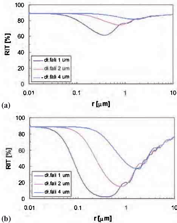
Rys. 9. RIT w funkcji promienia porów dla: a - V_p = 1 \times 10^{-4} , b - V_p = 1 \times 10^{-3} , grubość próbki 1 mm. Fig. 9. RIT versus the pore radius. Porosity: a - V_p = 1 \times 10^{-4} , b - V_p = 1 \times 10^{-3} , sample thickness - 1 mm.
