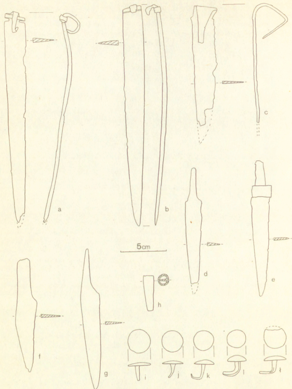
Ryc. 11. Pikule, gm. Janów Lubelski, stan. 2. Przedmioty żelazne z obiektu 7 (a) oraz z obiektów o nie ustalonej lokalizacji (b—f):
