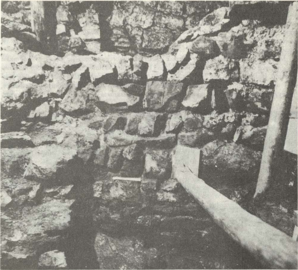
Ryc. 2. Kraków-Wawel. Dziedziniec Batorego, wykop 2/70–83. Wątek lica fundamentu zachodniej ściany kościoła św. Gereona
