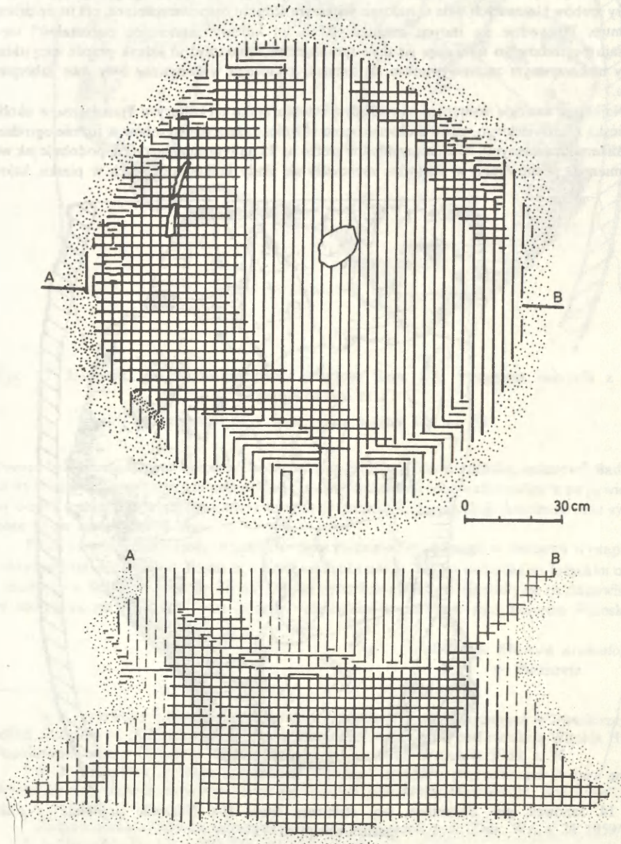
Ryc. 13. Janówek, gm. Skrzyszew, woj. stołeczne. Stan. I/A. Plan i profil pieca garncarskiego, obiekt nr 71
