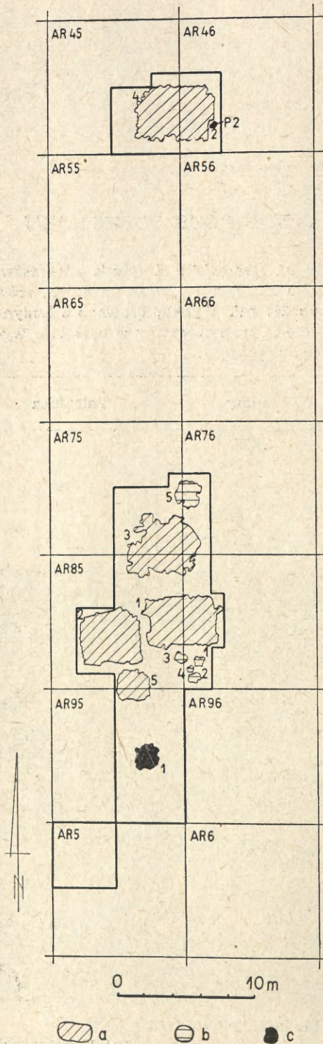
Ryc. 2. Piwonice, pow. Kalisz. Plan odcinka stanowiska 1, przebadanego w 1965 r. a — budynki; b — jamy; c — paleniska kamienne
