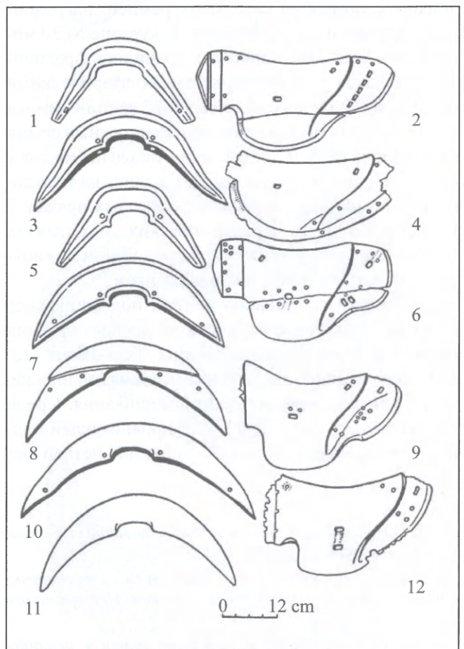
Рис. 8. Седла древних тюрков Саяно-Алтая: 1-3 – Кокэль, к. 2; 4, 8, 11 – к. 23; 5-7 – к. 22; 9 – к. 47; 10, 12 – к. 6.
