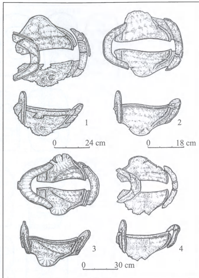
Рис. 4. Седла древних тюрков Тянь-Шаня: 1 – Беш-Таш-Короо II, к. 30; 2 – к. 35; 3 – к. 39; 4 – к. 20.
