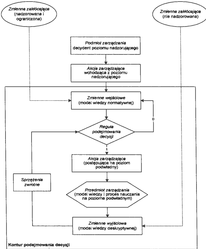
Rysunek 2. Struktura konturu zarządzania Otwartego Systemu Nauczania Zdalnego (OSNZ)
