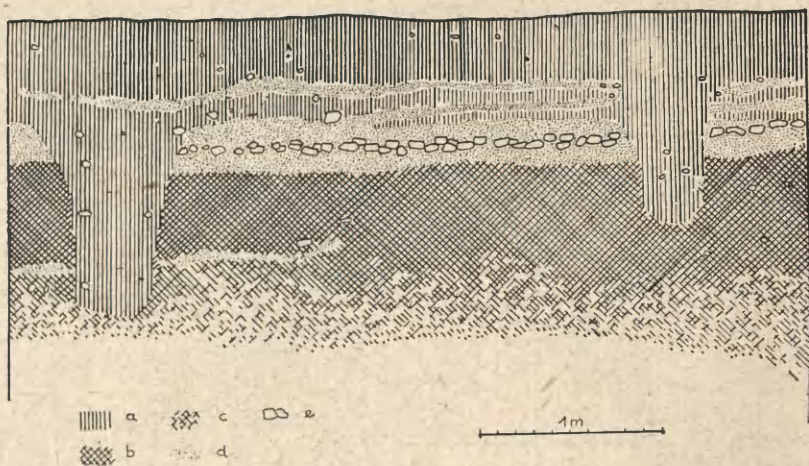
Ryc. 5. Chroberz, pow. Pińczów, stan. 1. Profil główny nawarstwień kulturowych:
