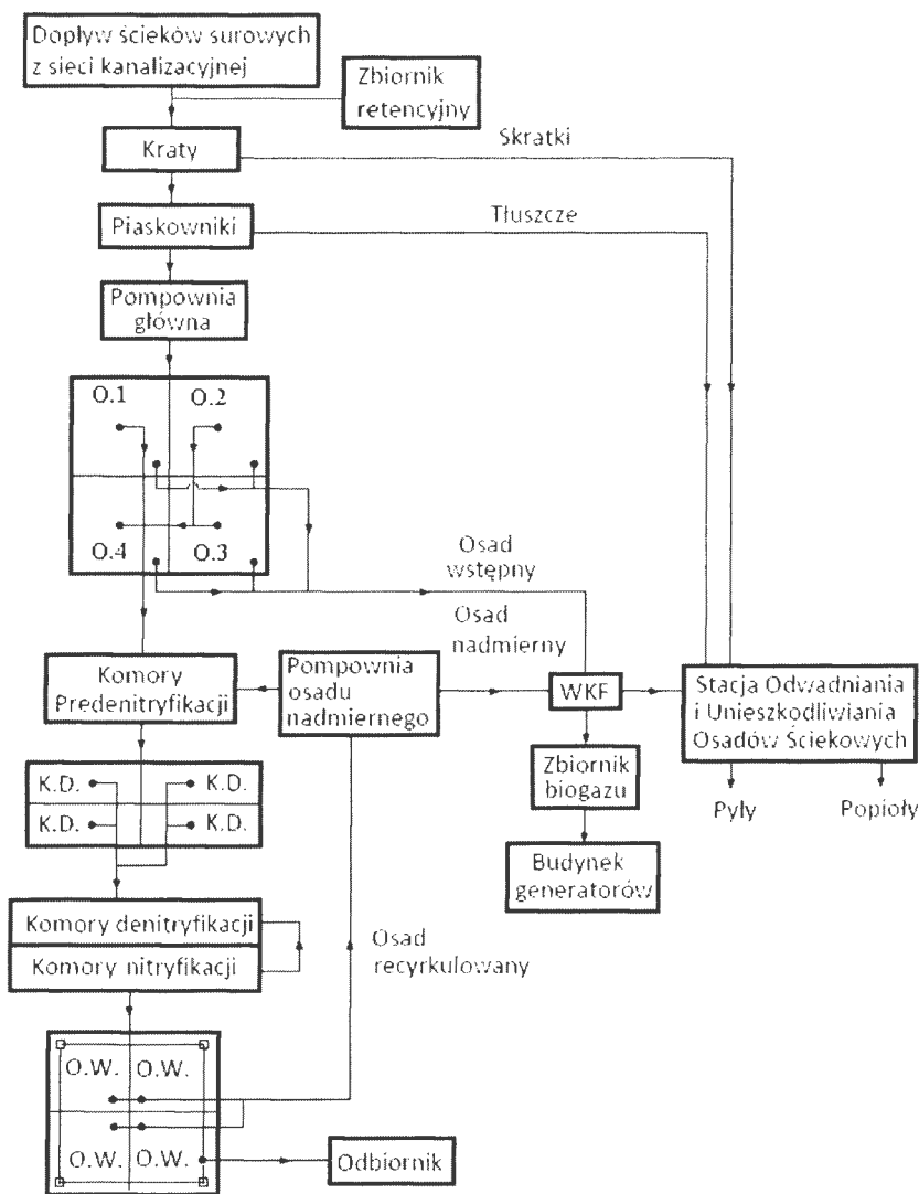
Rys. 4.1. Schemat oczyszczalni ścieków w Sitkówce-Nowiny.
