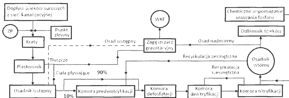
Rys. 4.2. Schemat technologiczny oczyszczalni w Trepczy.
