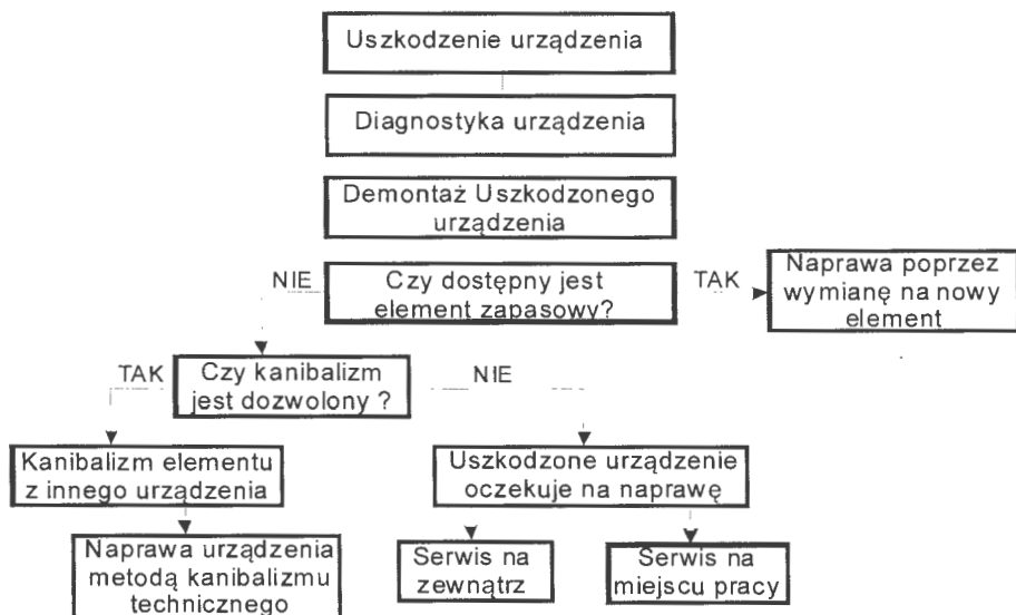
Rys. 2. Idea procedury naprawy urządzenia z możliwością zastosowania metody kanibalizmu technicznego
