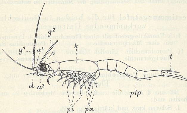
Fig. 485*). Mysis relicta Lovén ♀. a^1 erste Antenne, g^1 ihre Geißeln; a^2 zweite Antenne, g^2 ihre Geißel, d ihre Deckschuppe; o Auge; k Kopsbrustschild; pi Innenäste der Spaltfüße, pa ihre Außenäste; plp Pleopoden = Abdominalfüße; t Telson. (Nach Sars. Vergr. 4 : 1.)
