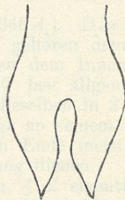
Fig. 345. Schwanzende von Argulus coregoni .
