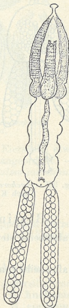
Fig. 332. Tracheliastes polycolpus (nach Nordmann.)
