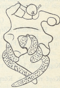
Fig. 343. Diocus gobinus (nach Steinstrup und Lütken).
