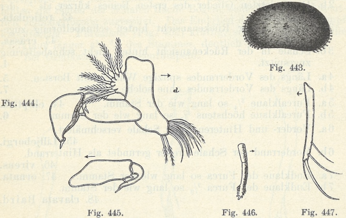
Fig. 443. Cypris incongruens Ramd. in der Seitenansicht. — Fig. 444. Kieferfuß der rechten Seite. — Fig. 445. Taster des Kieferfußes der linken Seite. — Fig. 446. Eine Klaue der 1. Maxillarlade. — Fig. 447. Furca.
