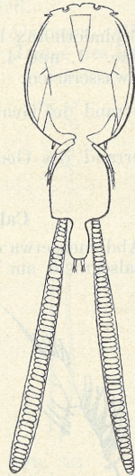
Fig. 317. Caligus lacustris (n. Steenstrup u. Lütken).
