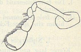
Fig. 503 nach Bate; Vergr. 11:1.
