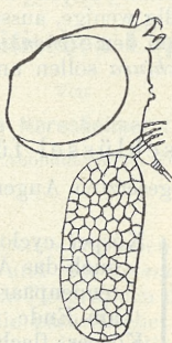
Fig. 313. Ergasilus gasterostei (nach Kr.)
