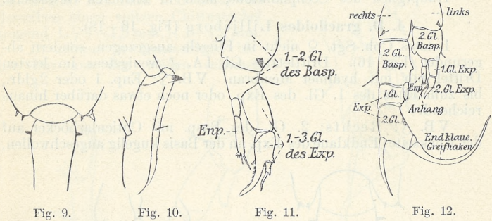
Fig. 9—12. Diaptomus Zachariae Poppe. — Fig. 9. Letztes Ceph.-Sgt. und 1. Abd.-Sgt. ♀. — Fig. 10. Drittleztes Gl. IA. ♂. — Fig. 11. VB. ♀. — Fig. 12. VB. ♂. (Nach Schmeil.)
