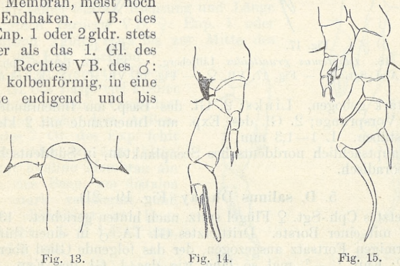
Fig. 13—15. Diaptomus gracilis O. Sars. — Fig. 13. Letztes Cph.-Sgt. und 1. Abd.-Sgt. ♀. — Fig. 14. VB. ♀. — Fig. 15. VB. ♂. (Nach Schmeil.)
