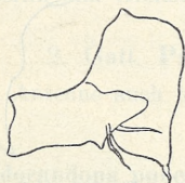
Fig. 384. Candona Bradyi Hartw. Rechtes Greiforgan des ♂.
