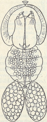
Fig. 329. Achtheres percarum (n. Nordmann).
