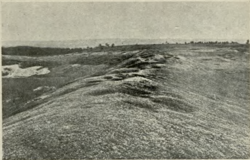
Oz (wał podlodowcowy) „Góra Szyszkina“ za przedmieściem Śnipiszki.
