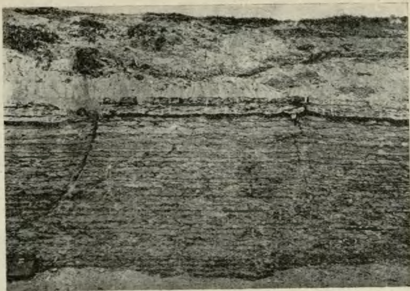
Potęźna serja ilów uwarstwionych, przykryta piaskami. (Zakret pod Wilnem).
