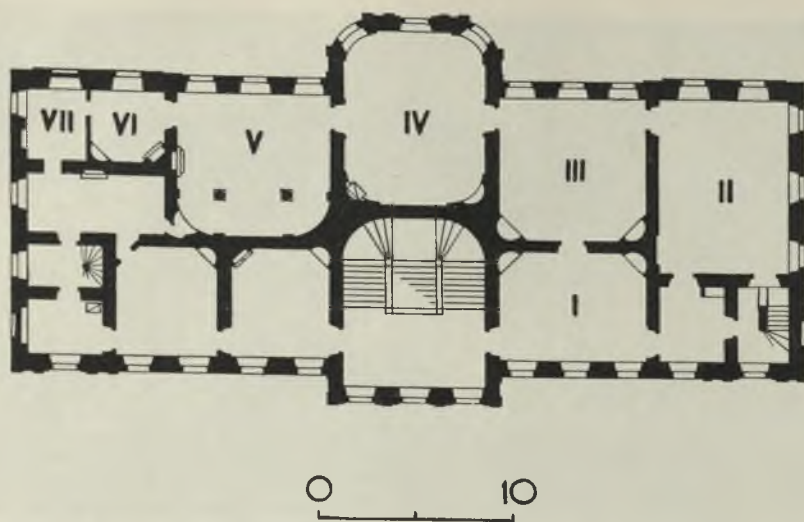
Ryc. 3. Świack. Rzut I. piętra pałacu.
