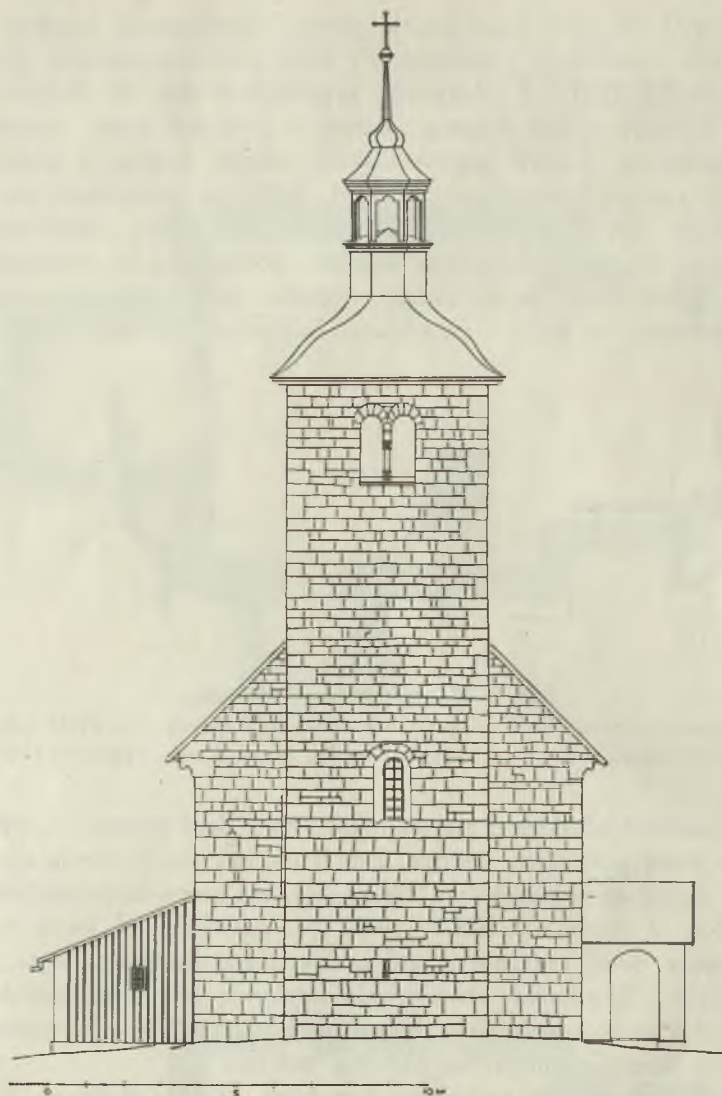
Ryc. 6. Wysocice. Kościół parafjalny. Elewacja zachodnia.
