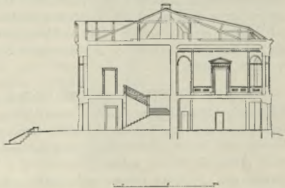
Ryc. 8. Świack. Przekrój poprzeczny pałacu.
