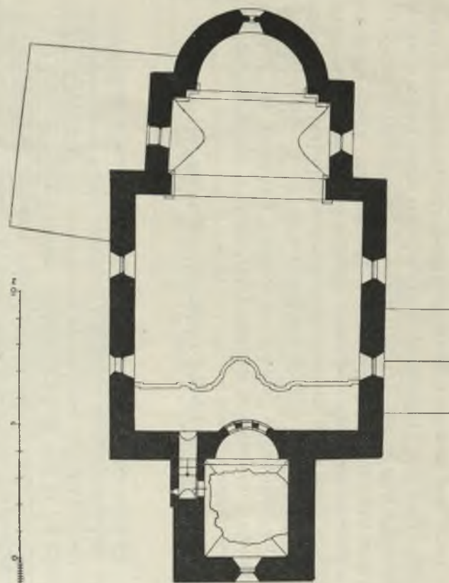
Ryc. 4. Wysocice. Kościół parafjalny. Rzut na wysokości okien.
