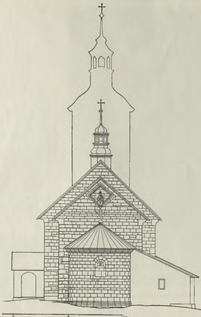
Ryc. 7. Wysocice. Kościół parafjalny. Elewacja południowa.
