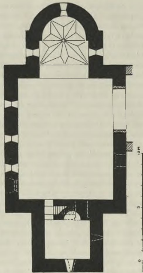
Ryc. 14. Kościelec. Kościół p. w. Przemienienia Pańskiego. Rzut poziomy.
