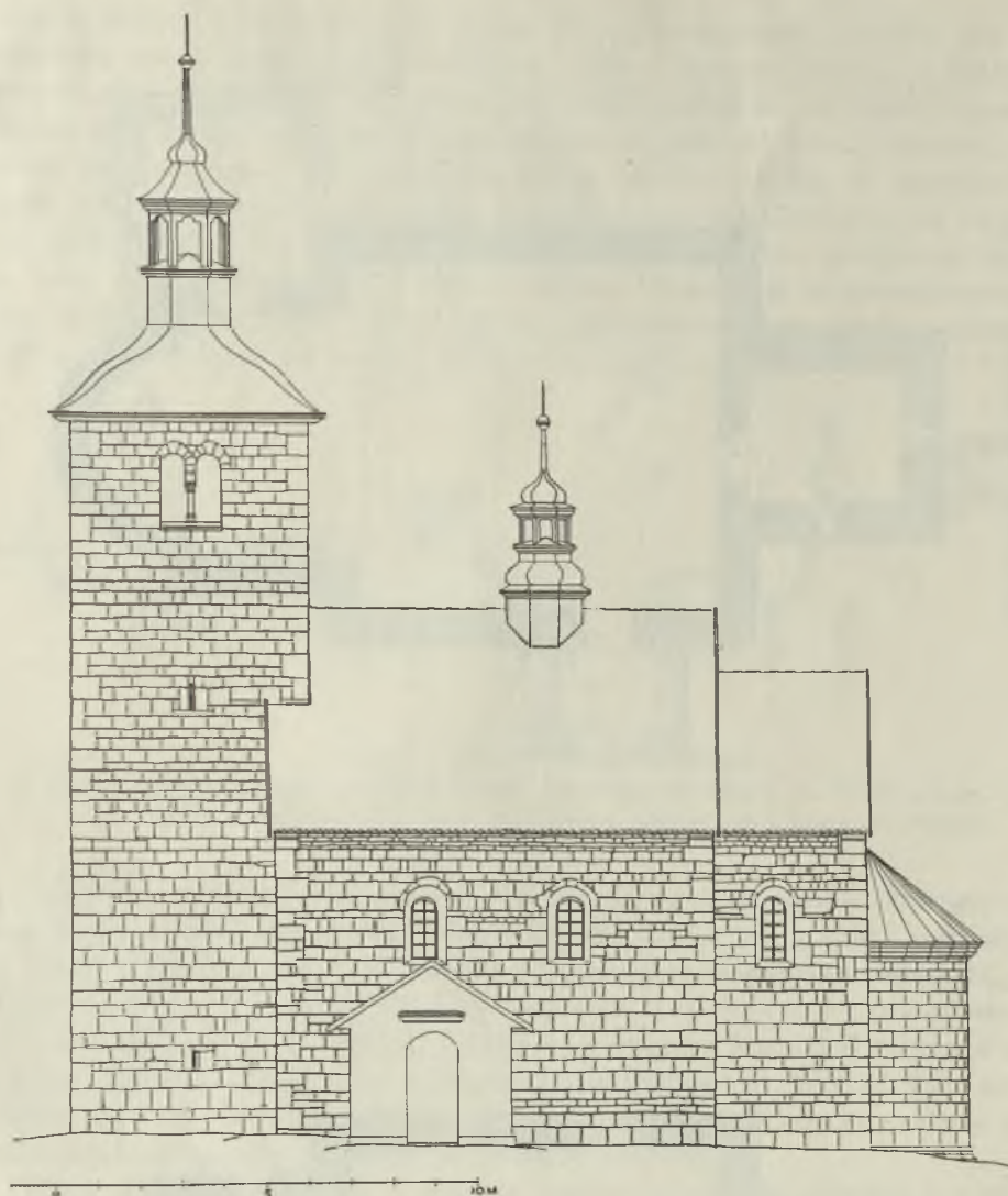
Ryc. 2. Wysocice. Kościół parafjalny. Elewacja południowa.
