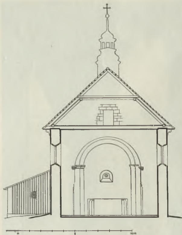
Ryc. 10. Wysocice. Kościół parafjalny. Przekrój poprzeczny.
