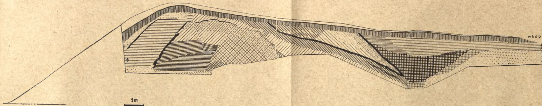
Ryc. 2. Myślibórz. Przekrój poprzeczny przez wał grodziska widziany od północy
