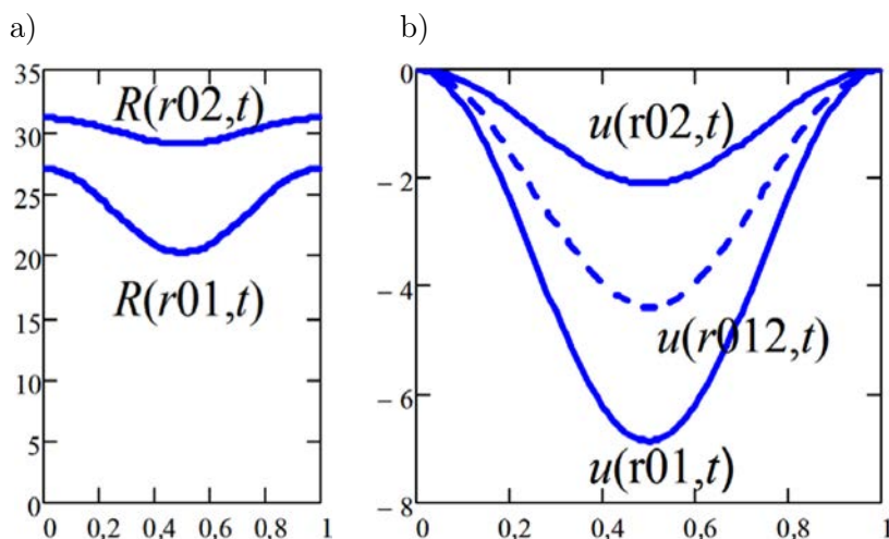
Rys. 6.2. a) Przebieg deformacji ściany w czasie pełnego cyklu; b) przebieg przemieszczenia granic ściany i środkowej warstwy wewnętrznej r = r_{012} = (r_{01} + r_{02})/2 (kreskowana linia niebieska). Oś pionowa wyskalowana w [mm], oś pozioma w jednostkach czasu.
