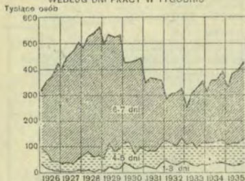
ZATRUDNIENI W PRZEMYSŁE PRZETWÓRCZYM WEDŁUG DNI PRACY W TYGODNIU
