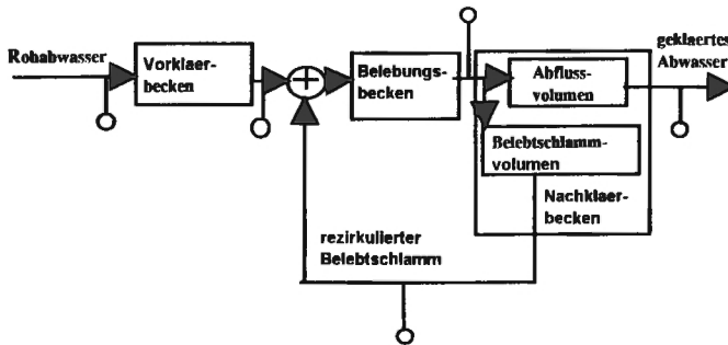
Abb. 2. Schaltbild der Hauptbehälter der Kläranlage in Rzeszow. Mit den Kreiszeichen sind die ausgewählten Meßstellen bezeichnet (Abfluss- bzw. Belebtschlammvolumen bedeutet Klär- bzw. Sedimentationszone der Nachklärbecken)
