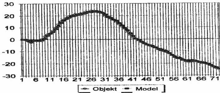
Abb. 9. Meß- und Rechenwerte für die Sedimentationszone der Nachklärbecken; a - und b -Einschätzung.
