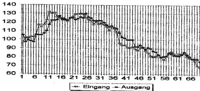
Abb. 4. Meßwerte für die Belebungsbecken.
