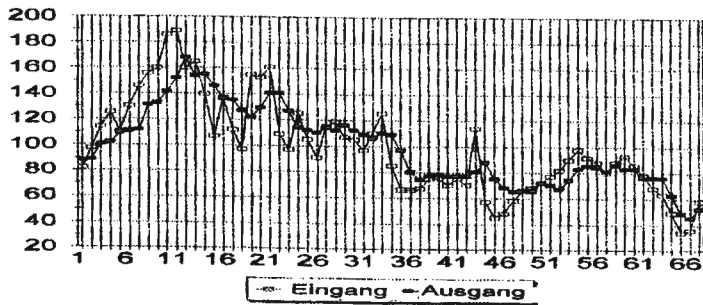
Abb. 3. Meßwerte für die Vorklärbecken.
