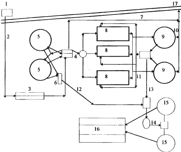
Abb. 1. Schema der untersuchten Kläranlage; 1 - Pumpenwerk, 2 - Rohabwasser, 3 - Sandbecken, 4 - Verteilungskammer, 5 - Vorklärbecken, 6 - Sammelkammer, 7 - Notabfluß, 8 - Belebungsbecken, 9 - Nachklärbecken, 10 - geklärtes Abwasser, 11 - rezirkulierter Belebtschlamm, 12 - Rohschlamm, 13 - Überbelebtschlamm, 14 - Schlammverdicker, 15 - Fermentationskammern, 16 - Schlammfelder, 17 - der Fluß.
