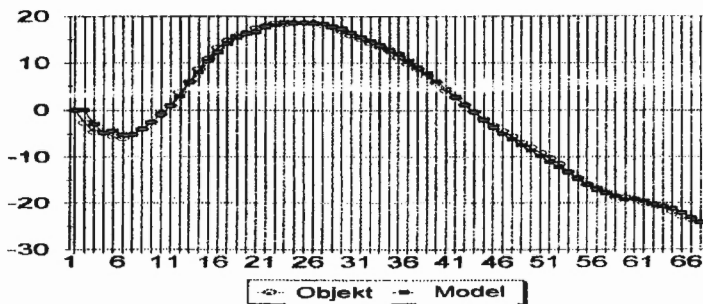
Abb. 10. Meß- und Rechenwerte für die Klärzone der Nachklärbecken; a - und b -Einschätzung.
