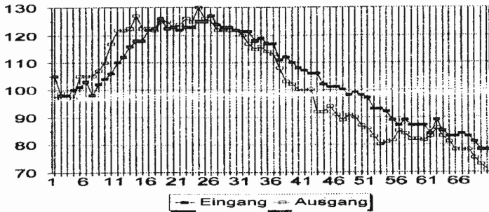
Abb. 6. Meßwerte für die Klärzone der Nachklärbecken.
