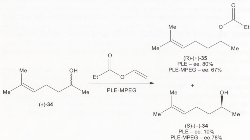
Rys. 13. Stereoselektywna transestryfikacja alkoholu drugorzędowego.
