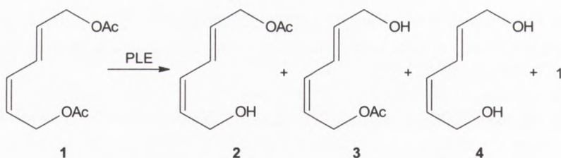
Rys. 2. Regioselektywna hydroliza estru dioli związku dienowego.
