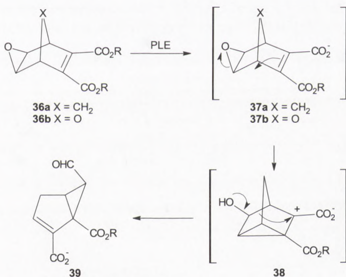
Rys. 14. Reakcja domino z przegrupowaniem Meinwalda.
