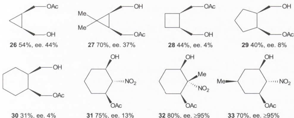
Rys. 12. Selektywna hydroliza estrów dioli.
