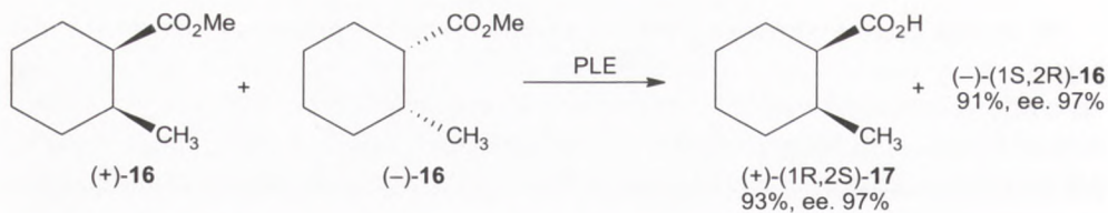
Rys. 7. Rozdział kinetyczny enancjomerów o konfiguracji cis .
