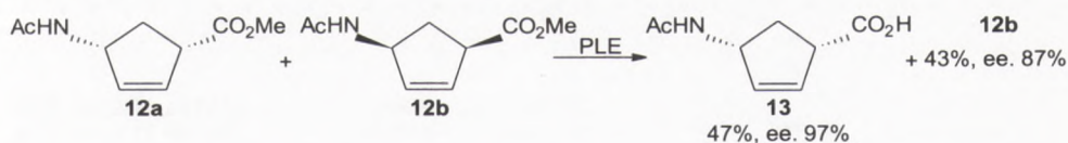
Rys. 5. Chemoselektywna hydroliza estrów.
