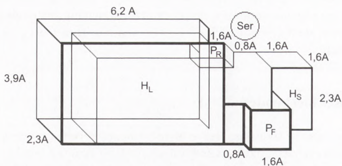
Rys. 1. Model centrum aktywnego esterazy wątroby wieprzowej wg Jonesa. H_L – duża i H_S – mała kieszeń wiążąca hydrofobowo. P_F – przednia i P_R – tylna kieszeń polarna. Ser – miejsce w którym występuje reszta serynowa triady katalitycznej.
