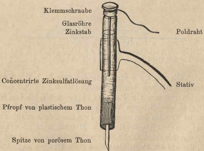
Eine unpolarisirbare, bewegliche Spitzenelektrode.
